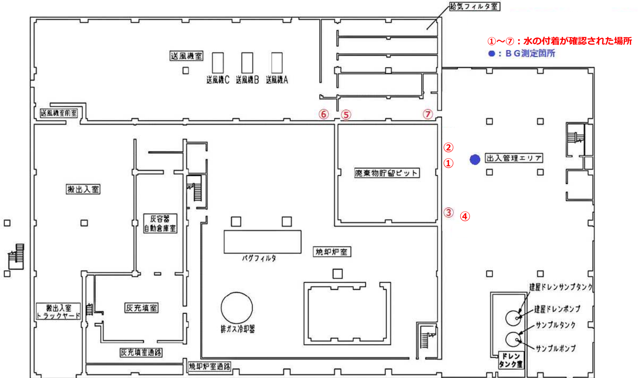
増設焼却炉建屋 1階
