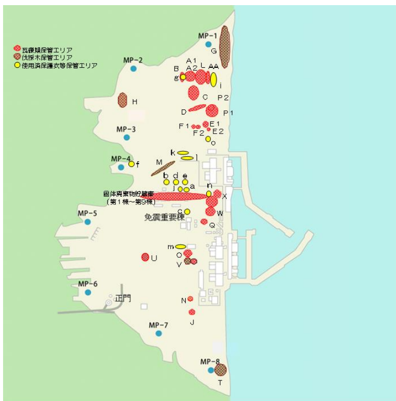
図 2.8-9 屋外一時保管エリア配置図
