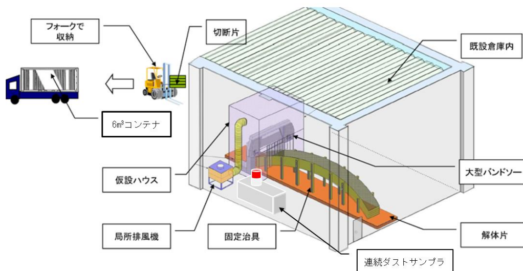
図 2.11-1 解体（減容）作業イメージ図
