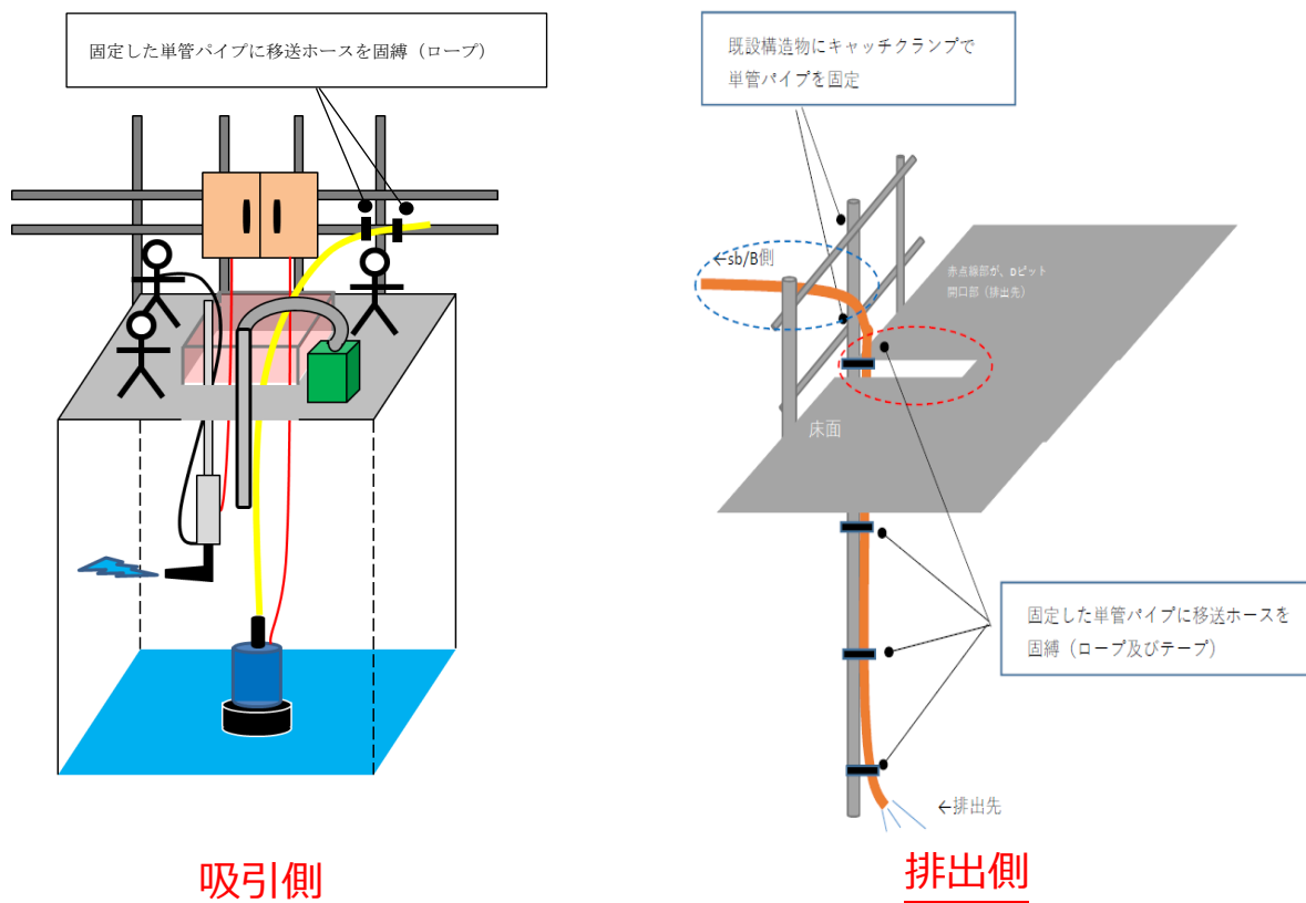
図 2.9-3 ホース固縛イメージ図
