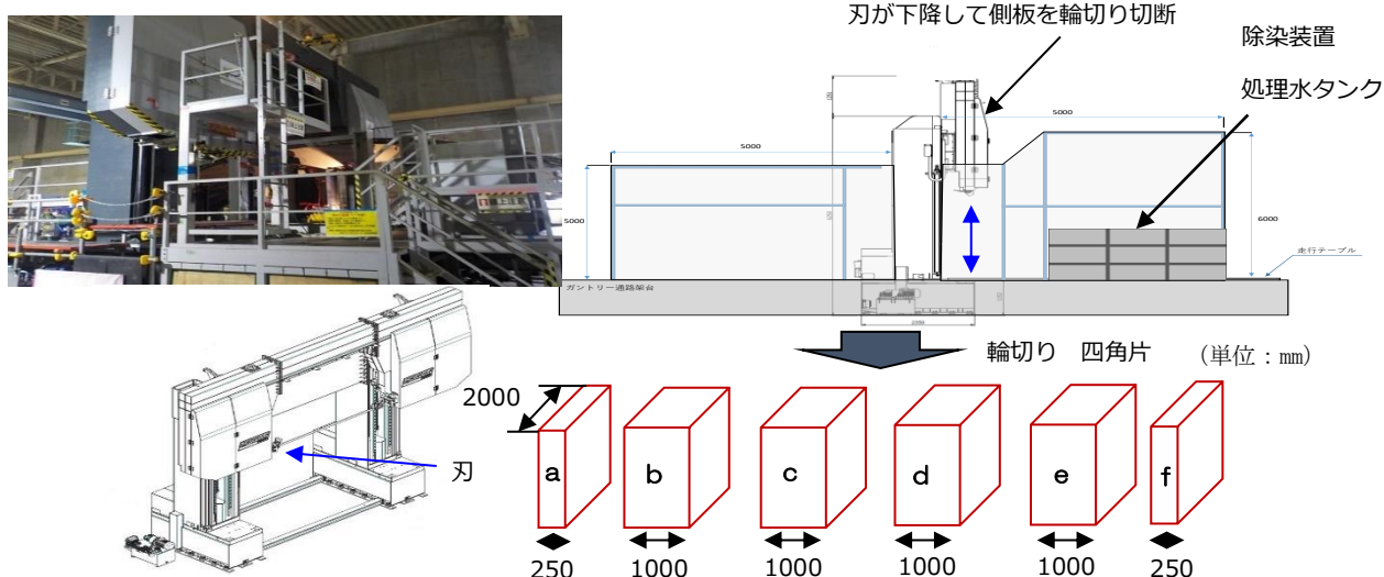
図 2.8-6 大型バンドソー輪切り切断イメージ図
