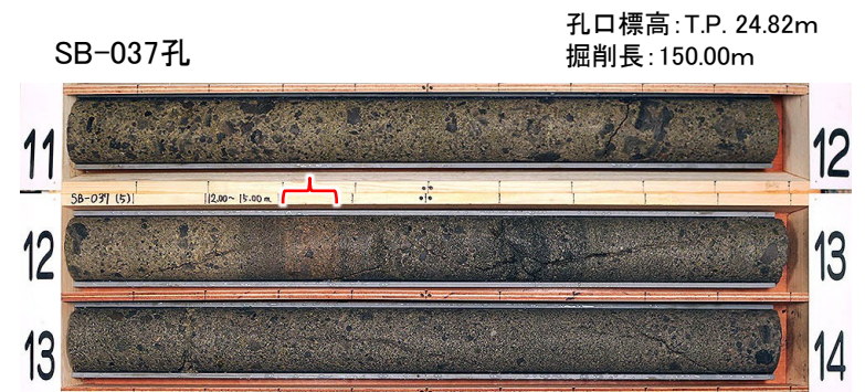
図5.24 SB-037孔コア写真
