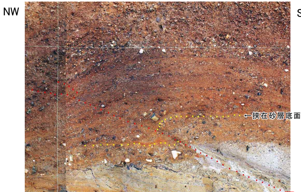
図1.4 法面詳細写真(Ts-6法面) 0 1m シーム S-11
