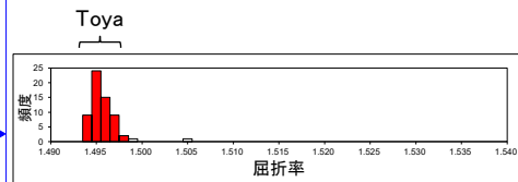
火山ガラス屈折率頻度分布
