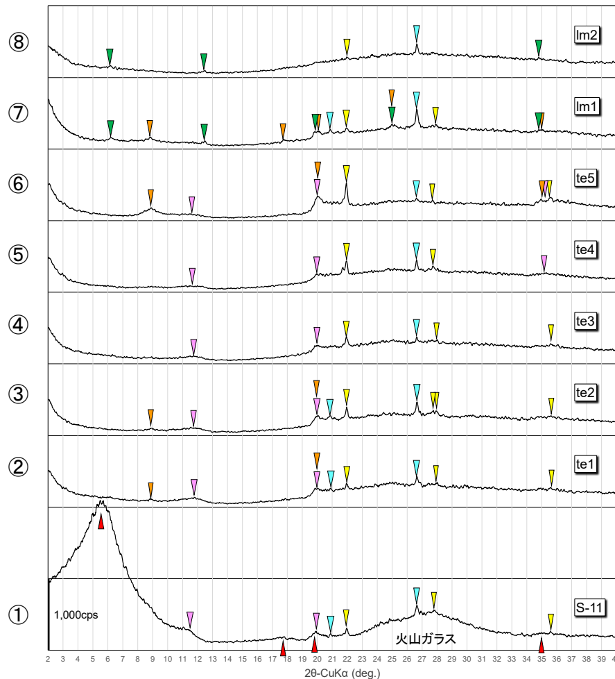
図4.3 シームS-11, その延長上のM 1 面段丘堆積物及びローム層の粉末X線回折分析結果
