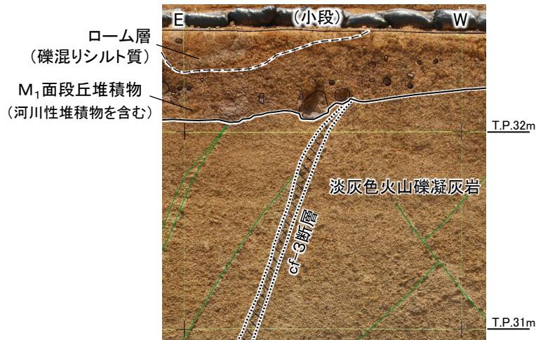
図3.3 Tf-5(a)トレンチ南側法面詳細写真(解釈線有り)
