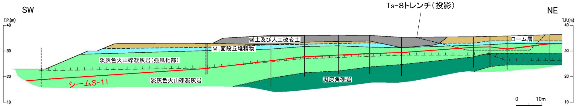
図1.20 Ts-8トレンチ付近地質断面図
