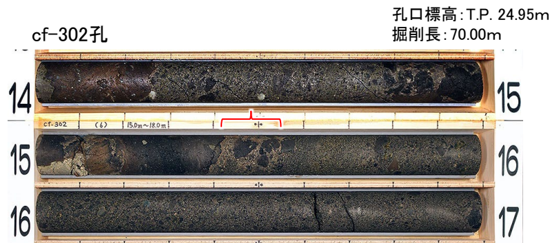
図5.23 cf-302孔コア写真
