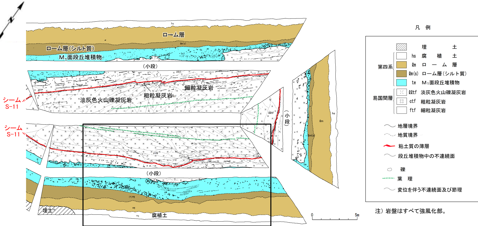
図5.25 Ts-8トレンチ全体スケッチ
