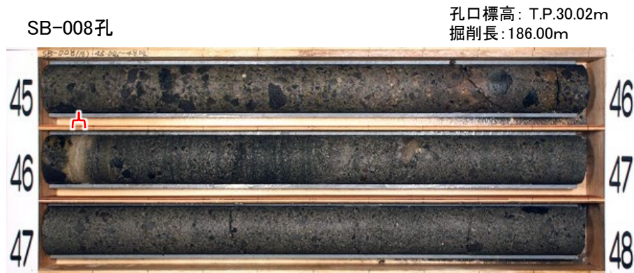
図5.17 SB-008孔コア写真
