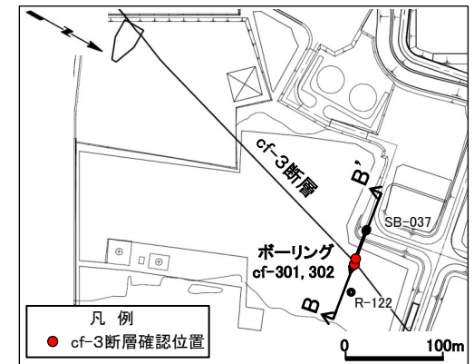
図5.20 断面位置図 注1) cf-3断層の分布はT.P.-14mにおける位置。
