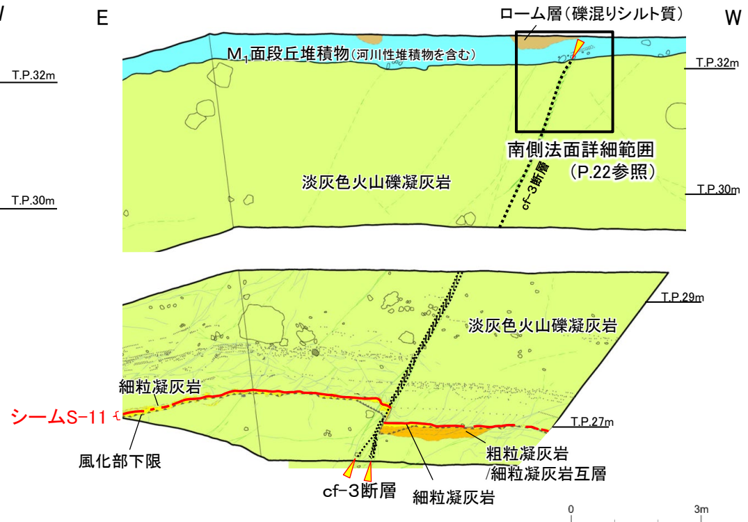
図3.2 Tf-5(a)トレンチ南側法面スケッチ
