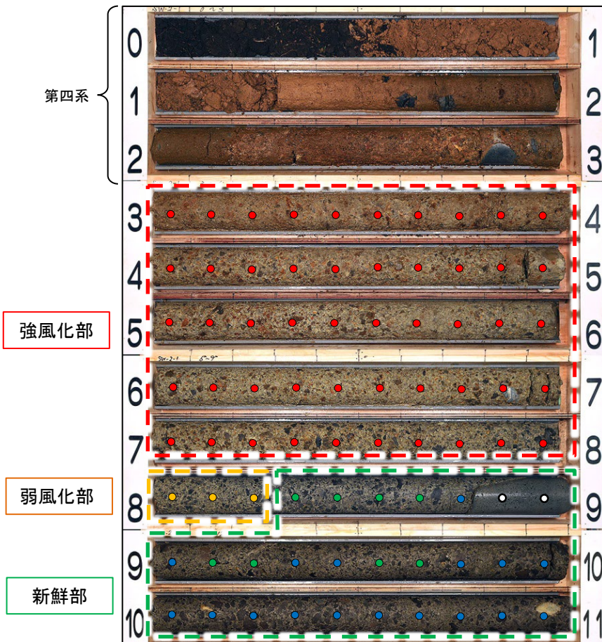
図1.22 易国間層(淡灰色火山礫凝灰岩)のボーリングコア(SW-2-1孔)での風化区分の例
