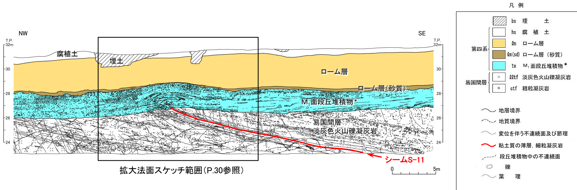
図5.2 M 1 面段丘堆積物に変位を及ぼしている箇所(Ts-6法面)
