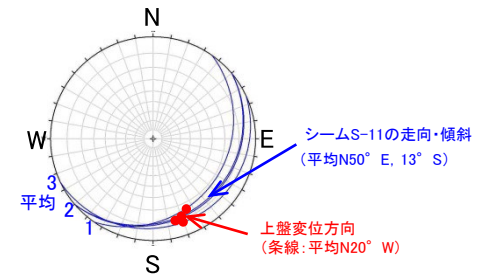
シームS-11の走向・傾斜及び上盤変位方向 (ウルフネット下半球投影)
