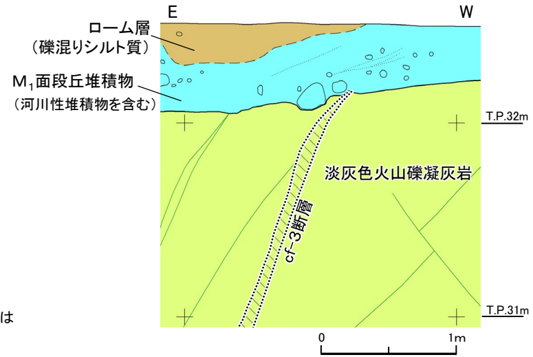
図3.5 Tf-5(a)トレンチ南側法面詳細スケッチ
