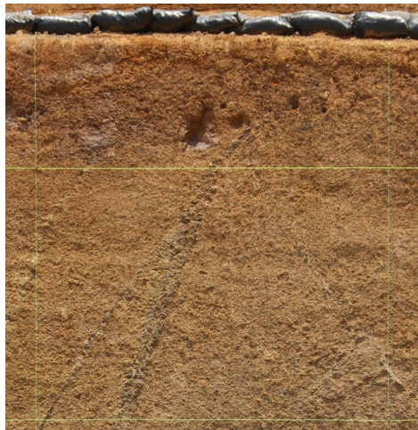
図3.4 Tf-5(a)トレンチ南側法面詳細写真(解釈線なし)
