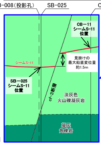
図5.2.13 断面拡大図
