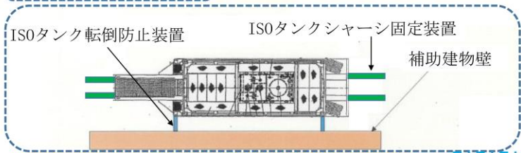
平面図（上から見た図）
