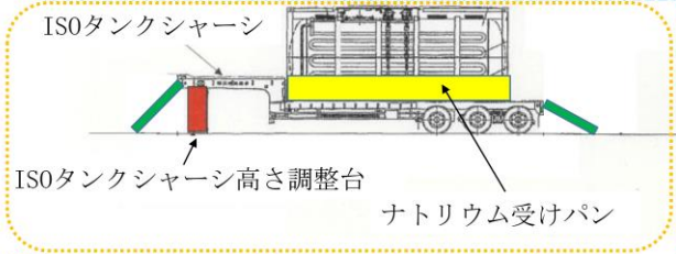
側面図（固定する補助建屋壁から見た図）
