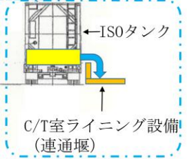
側面図（背後から見た図）
