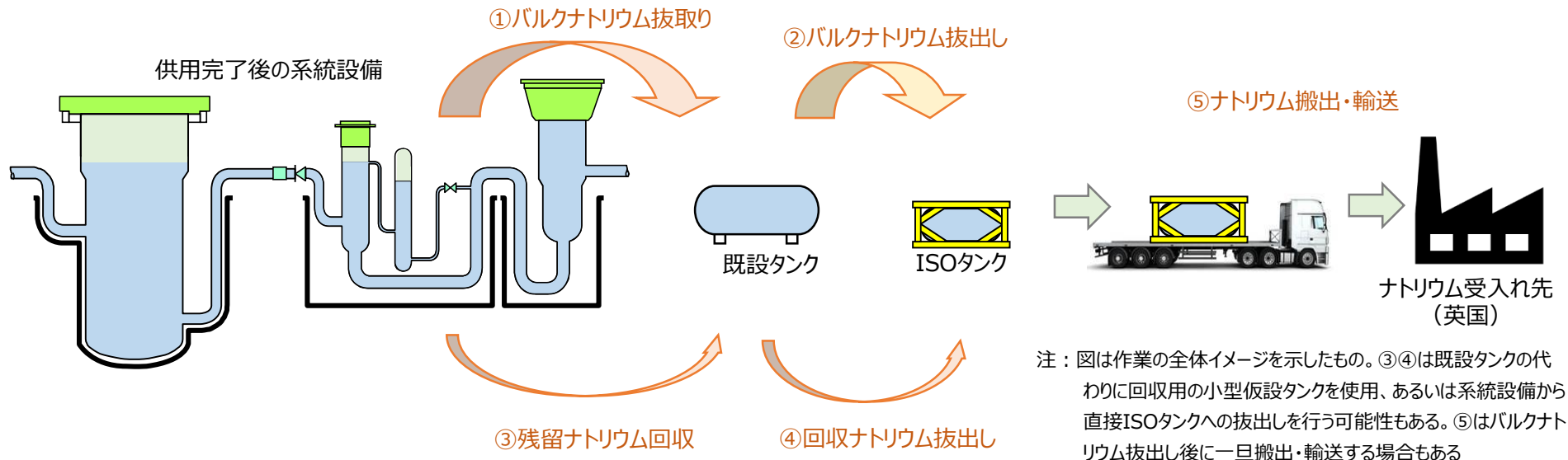
バルクナトリウム搬出までに必要な作業プロセス
