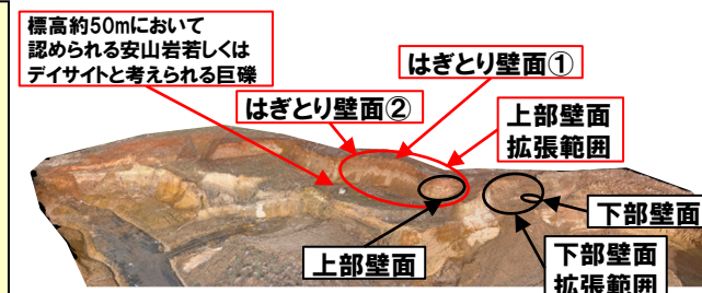
幌似露頭1付近の露頭状況写真 (南西方向から望む、令和5年12月当社撮影)
