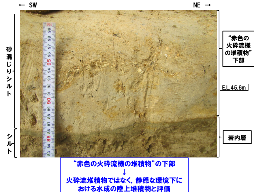
下部壁面拡大写真(令和5年8月撮影)
