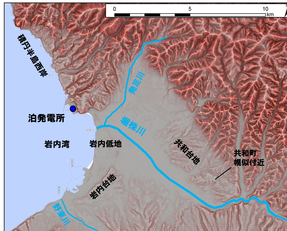
敷地及び敷地近傍の赤色立体地図
