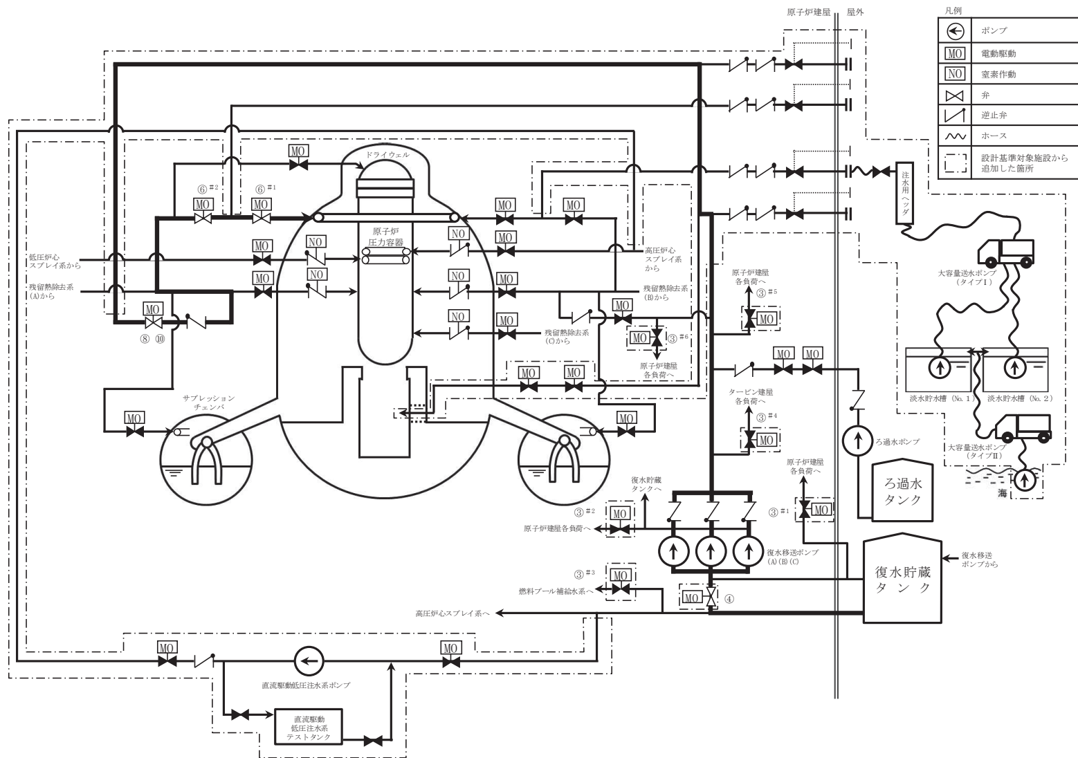
第 1.8-10 図 原子炉格納容器代替スプレィ冷却系（常設）による原子炉格納容器下部への注水 概要図（1/2）
