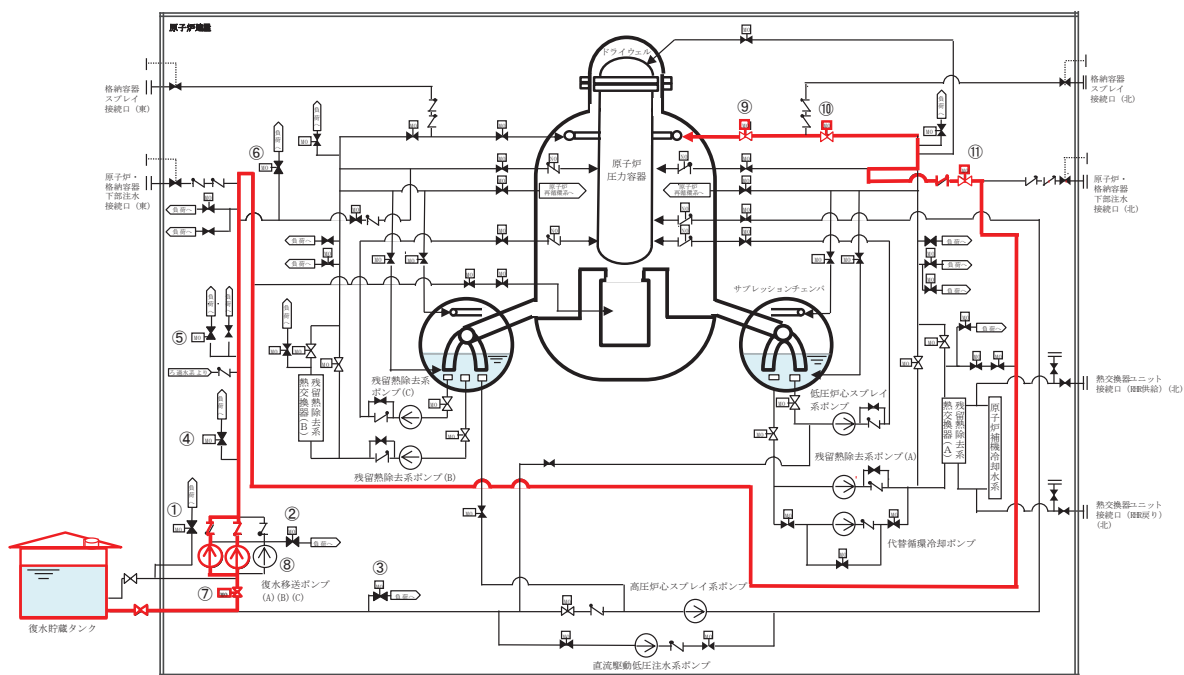
第3図 原子炉格納容器代替スプレィ冷却系（常設）による原子炉格納容器内へのスプレィ概略図
