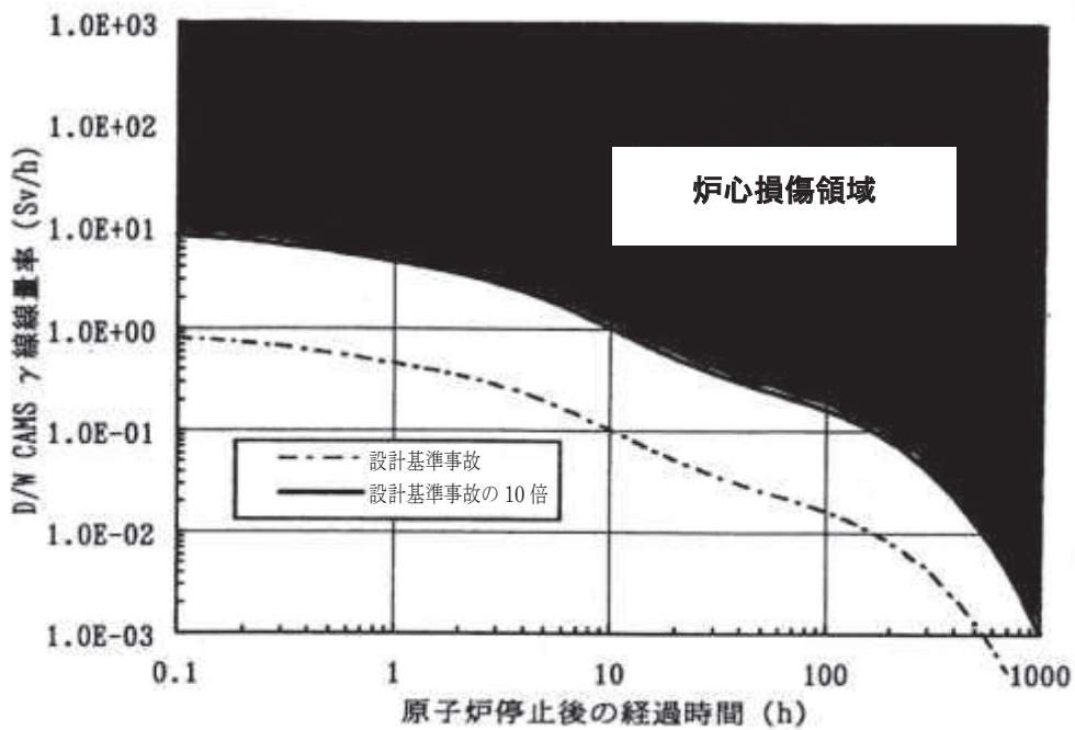
(1) ドライウエルのガンマ線線量率
