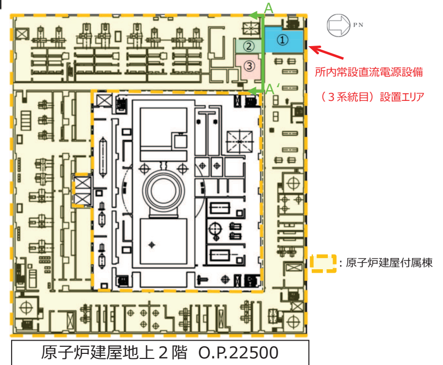
第 57-5-6 図 所内常設直流電源設備 (3系統目) 設置エリアと主な変更点
