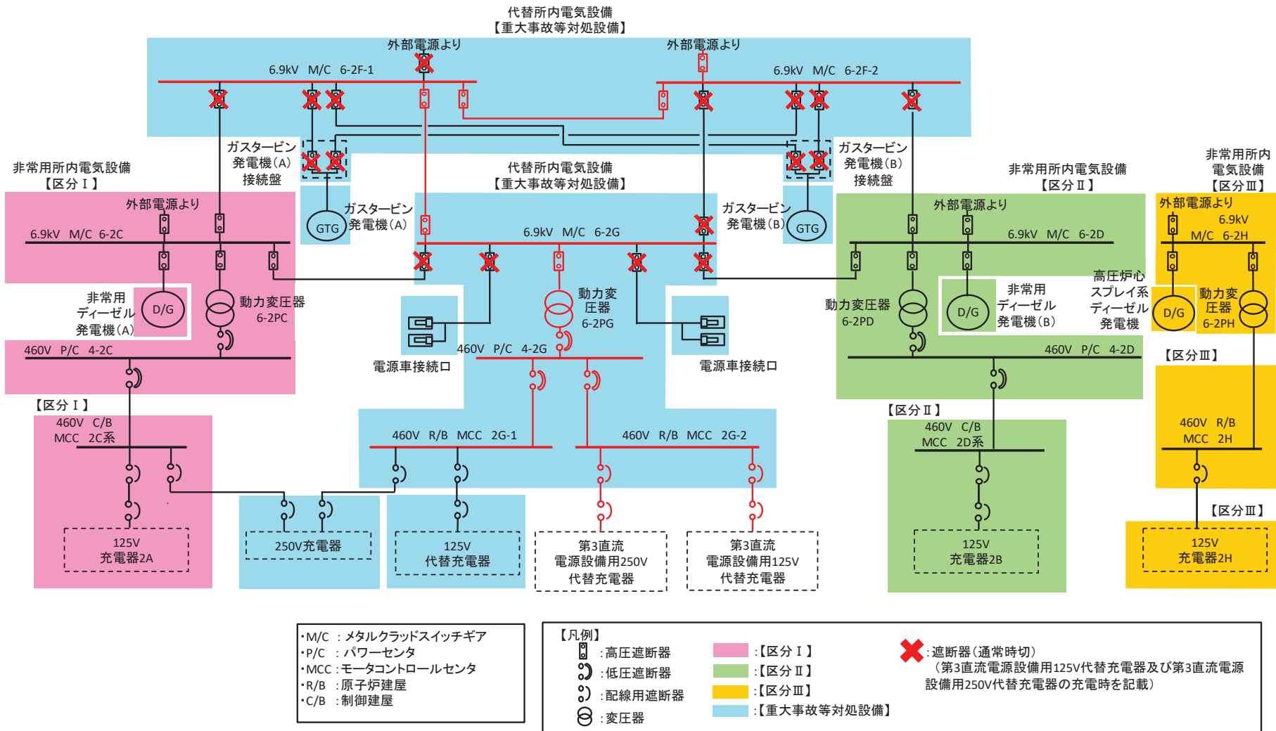
第 57-7-3-2 図 所内常設直流電源設備 (3 系統目) の受電系統図
