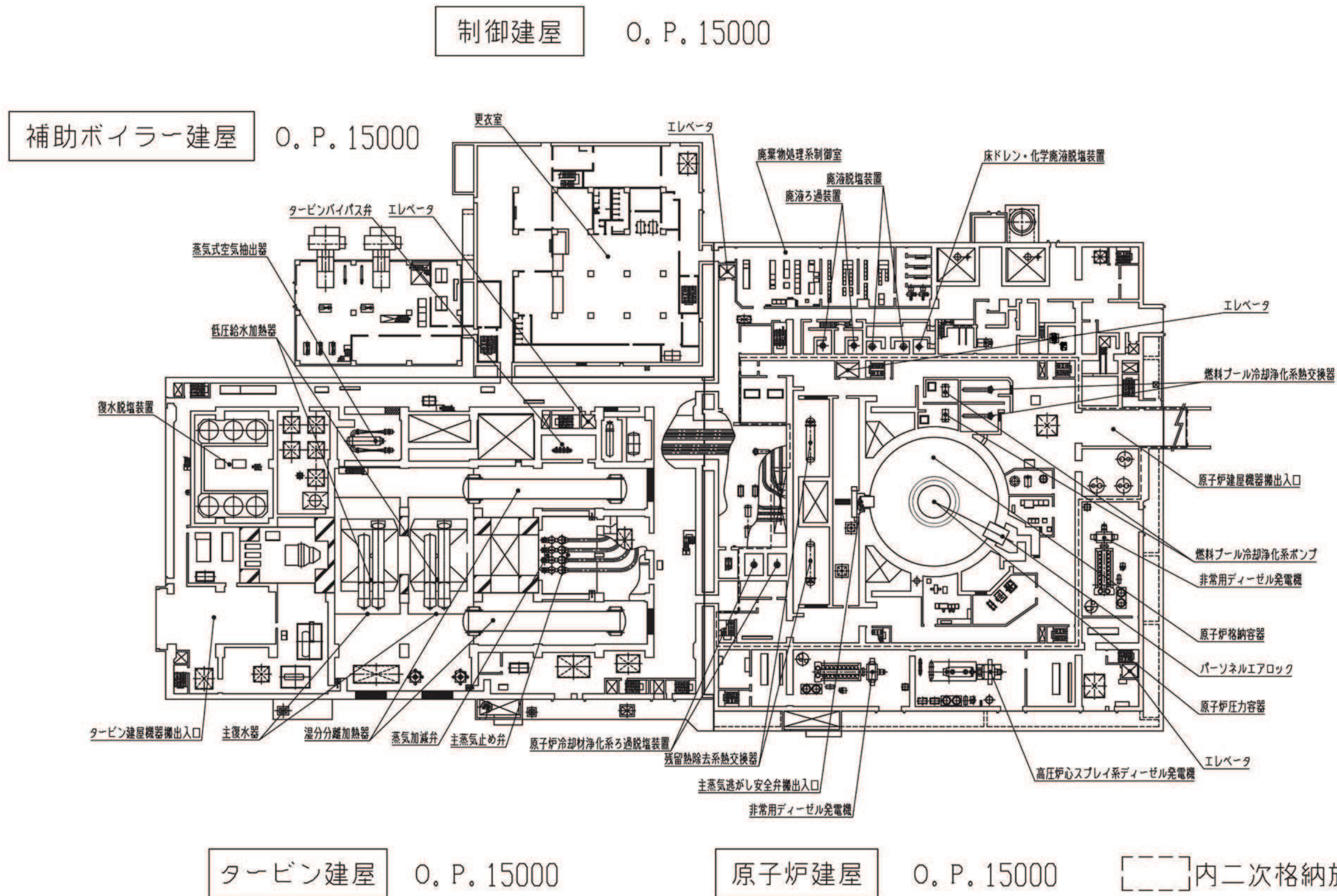
第 6 図 一階機器配置図
