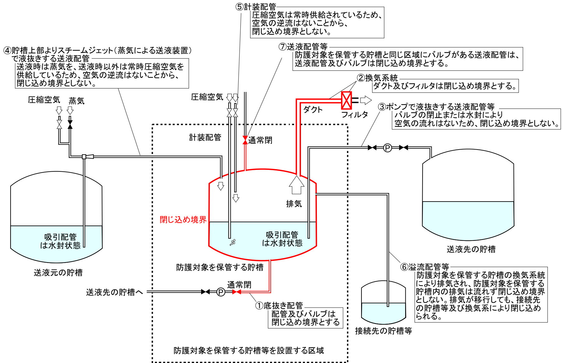
図-3 防護対象自体が液体の場合の閉じ込め境界に対する送液配管等の整理の概要
