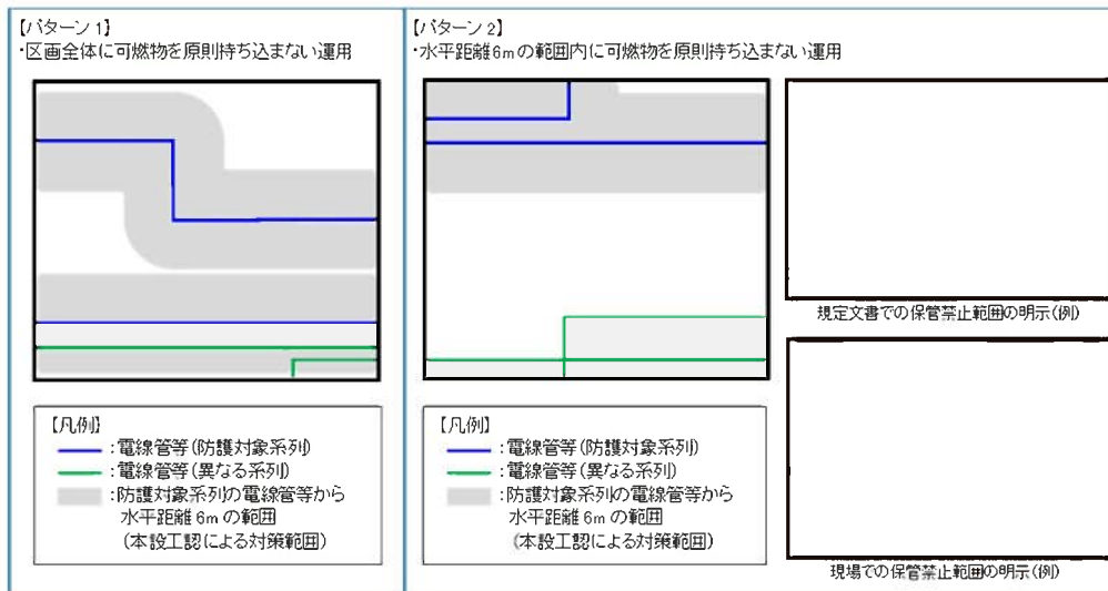
第 2 図 可燃性物質を原則持ち込まない運用とする範囲の具体例※
