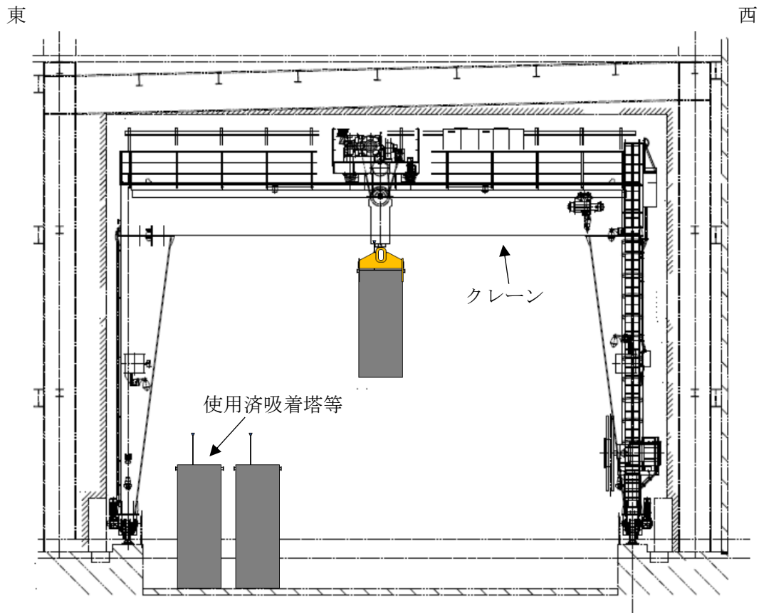
図 2-1 クレーンと使用済吸着塔の位置関係図
