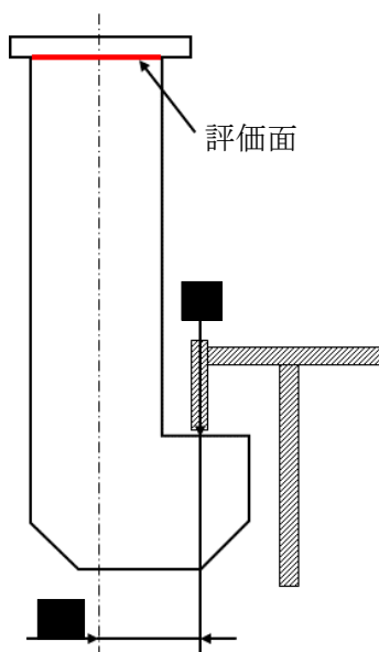
図 6-11 横行浮上り防止爪（根本）
