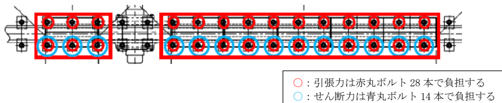
図 6-15 走行レールクリップ基礎ボルト
