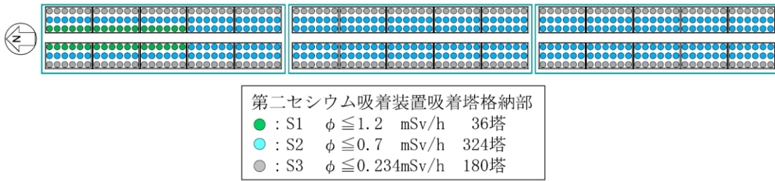
図－１ 大型廃棄物保管庫の吸着塔配置モデル（ \phi ：吸着塔側面線量率）（既認可） （実施計画：Ⅲ-3-2-2-2-添1-4）
