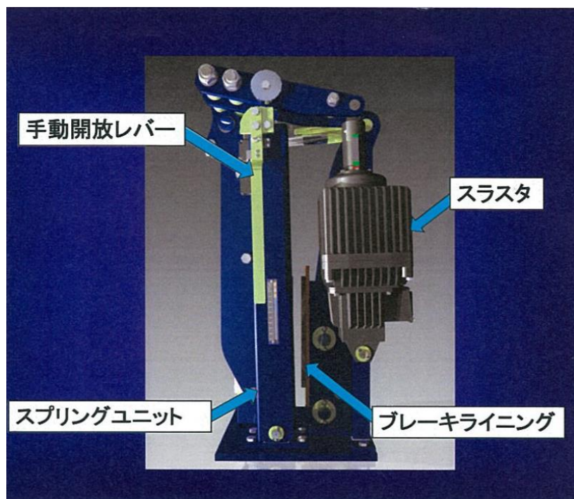
図－2 動力電源喪失時の吊荷落下防止策
