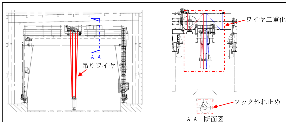
図－1 クレーンの吊荷落下防止策
