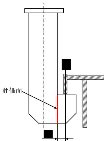
図 6-10 横行浮上り防止爪 (先端)
