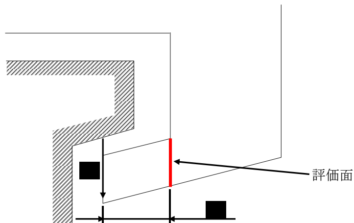
図 6-6 走行浮上り防止爪 (先端)
