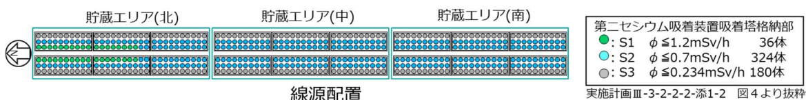
図-2 使用済吸着塔線源配置図
