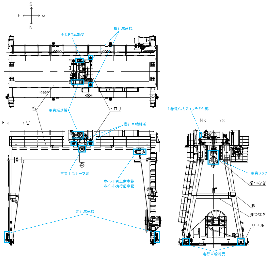
図-2 潤滑油を内包する構成部位
