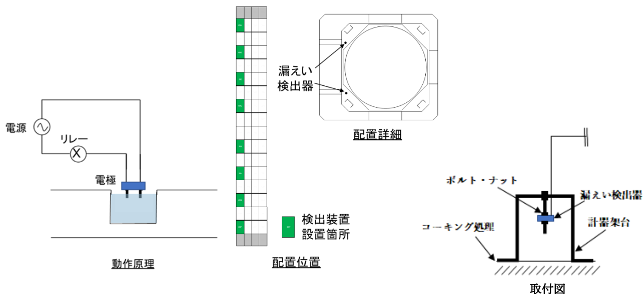
図 2.14.1-8 漏えい検出器の動作原理，設置状況
