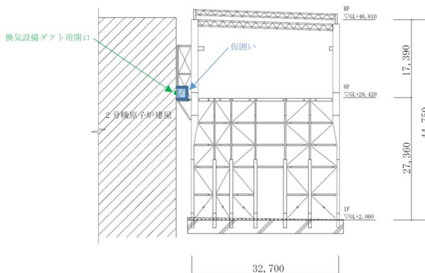
(2) 燃料取り出し用構台断面図 (1-1 断面)
