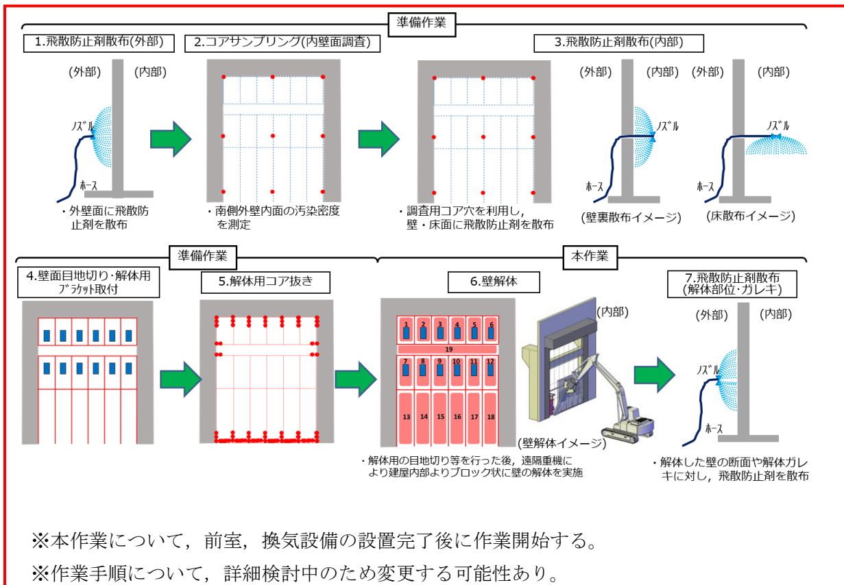
図3 ランウェイガード用開口における作業手順
