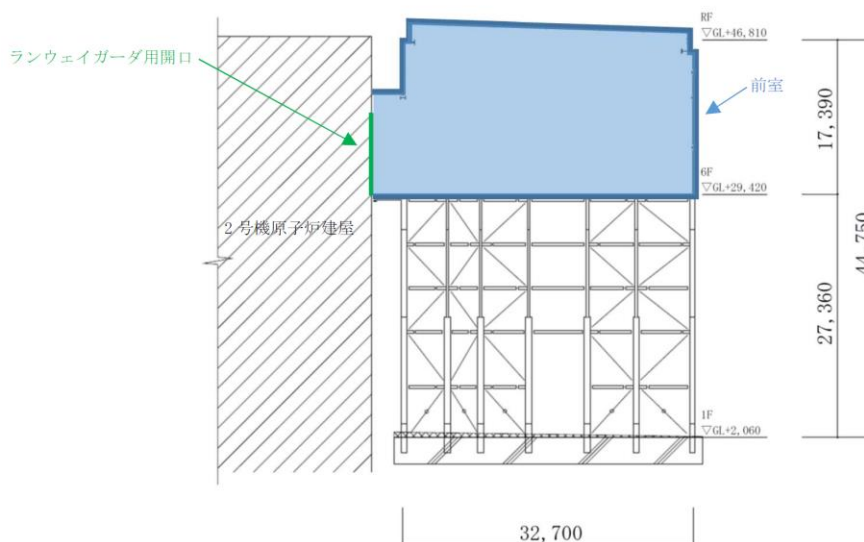
(2) 燃料取り出し用構台断面図 (2-2 断面)
