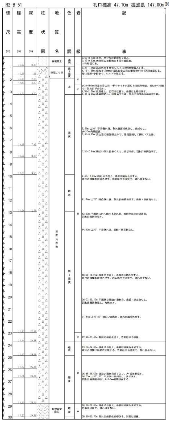
図 2.1.a.c-7 (9) 防潮堤（堀株側）ボーリング柱状図 R2-B-51 ボーリング (L=40m)
