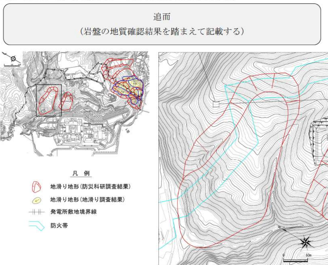
図 2.1.b.a-5 地滑り地形③分布図
