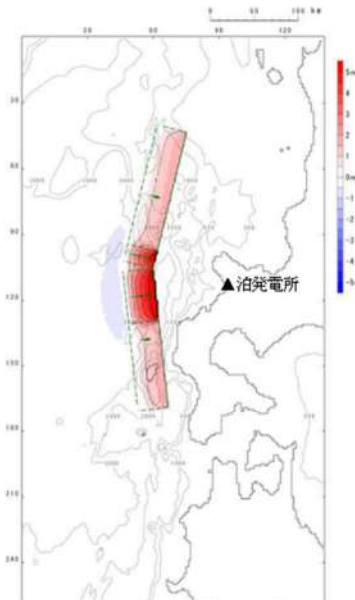
第 1.5-10 図（2） 地殻変動量分布図：最大隆起量発生波源
