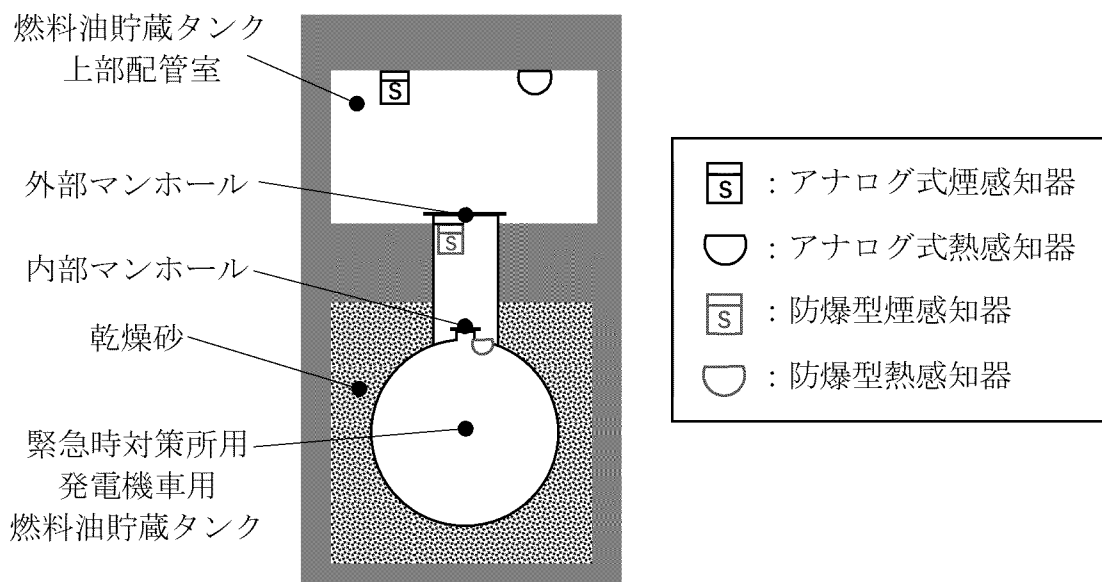
第 6-3-7 図 緊急時対策所用発電機車用燃料油貯蔵タンク室に対する火災感知器の 設置方法断面概要
