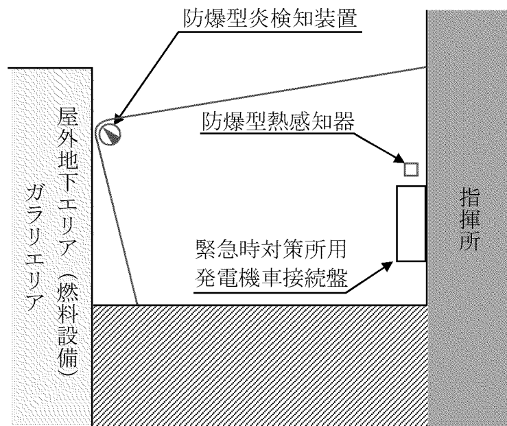
第 6-3-11 図 緊急時対策所用発電機車接続盤エリアに対する火災感知器の設置方法
