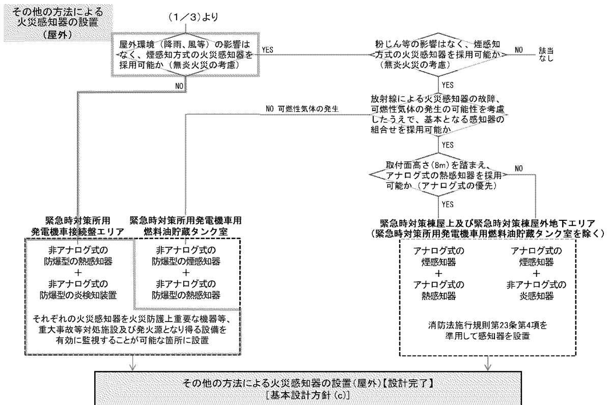
第 6-3-9 図 緊急時対策所用発電機車接続盤エリアの火災の感知の 設計フローにおける分類
