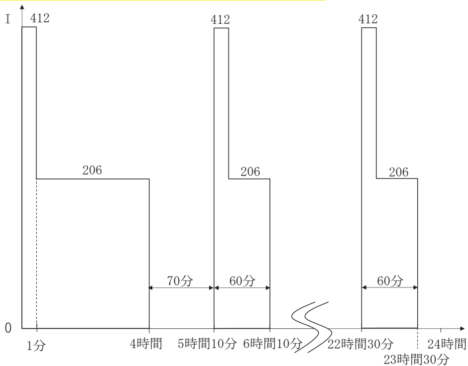
第 57-6-4 図 給電開始から 24 時間後までの負荷曲線
