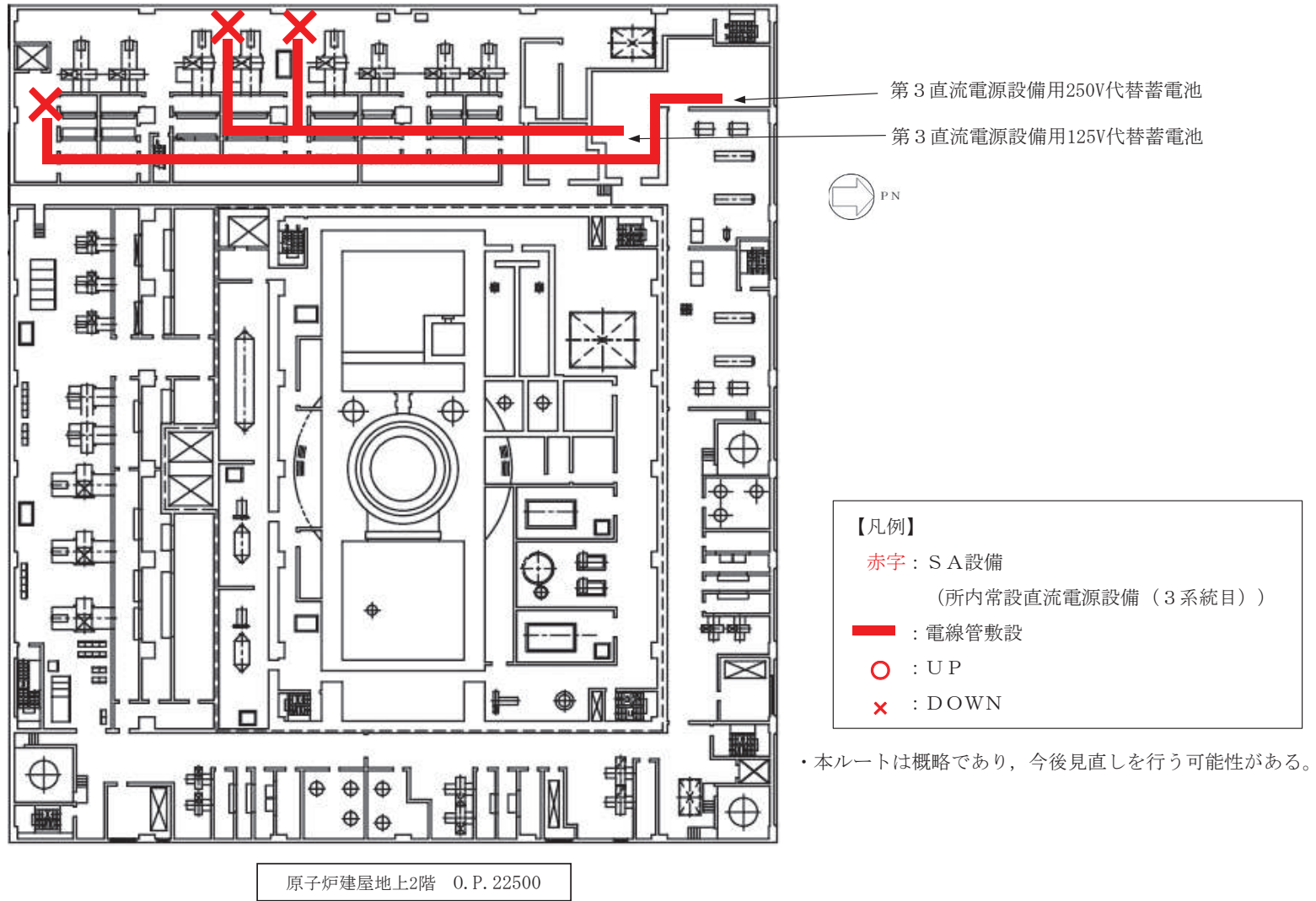
第 57-7-2-1 図 ケーブルルート図 (原子炉建屋地上 2 階)
