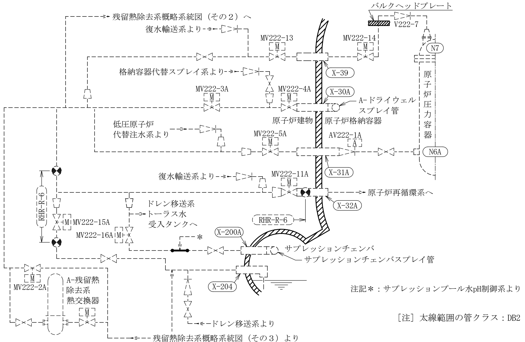
残留熱除去系概略系統図 (その1)
