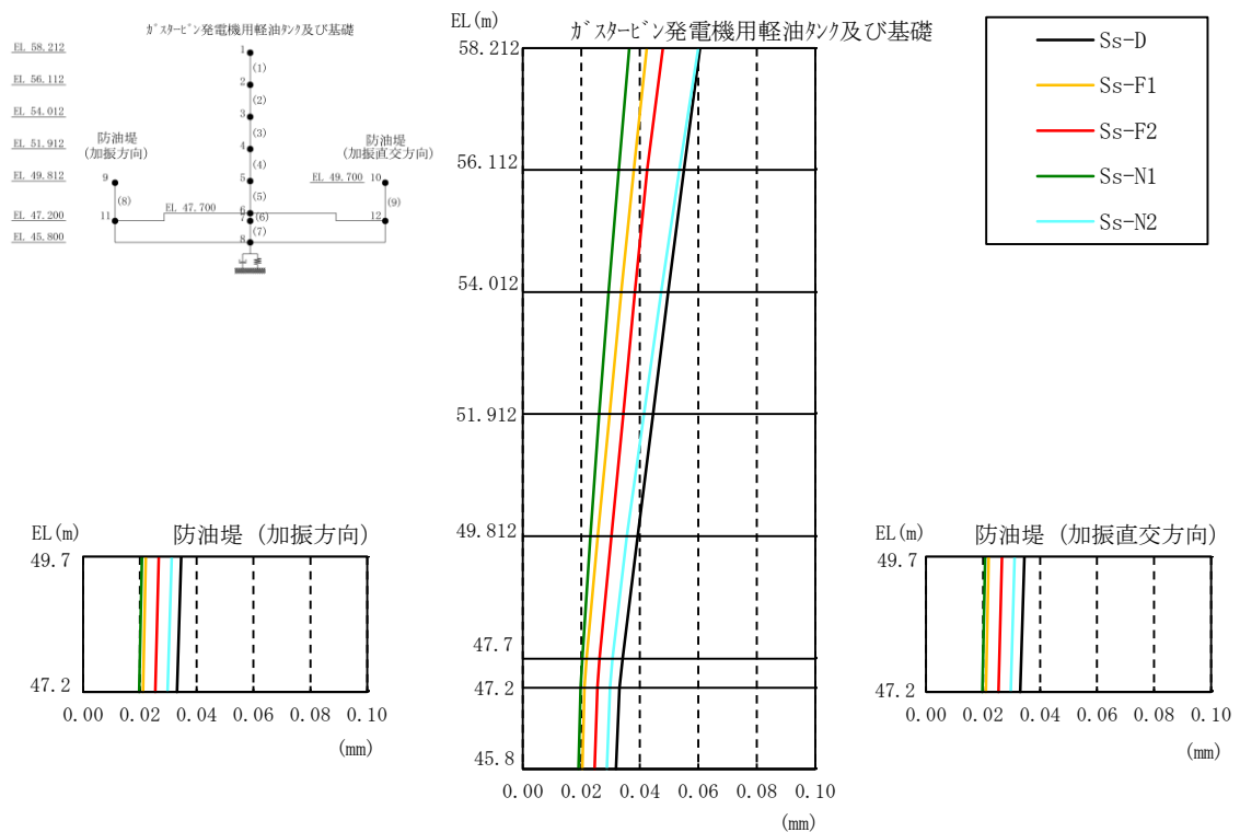
図 3-66 最大応答変位分布図（鉛直方向，解析ケース②）
