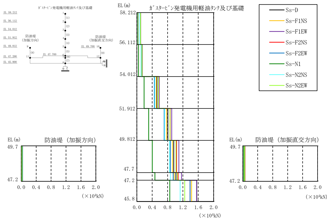
図 3-67 最大応答せん断力分布図（解析ケース②）
