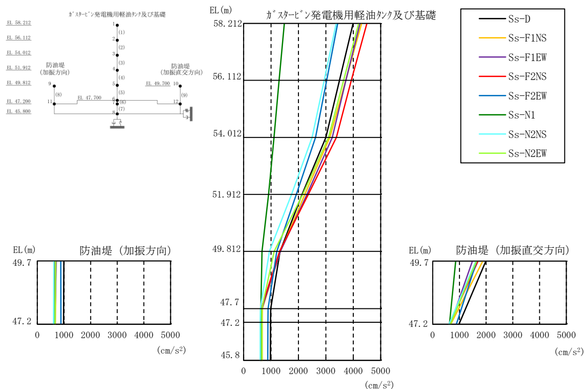
図 3-56 最大応答加速度分布図（水平方向，解析ケース①）
