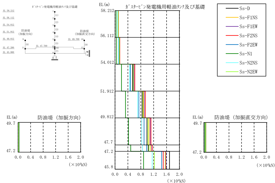
図 3-60 最大応答せん断力分布図（解析ケース①）
