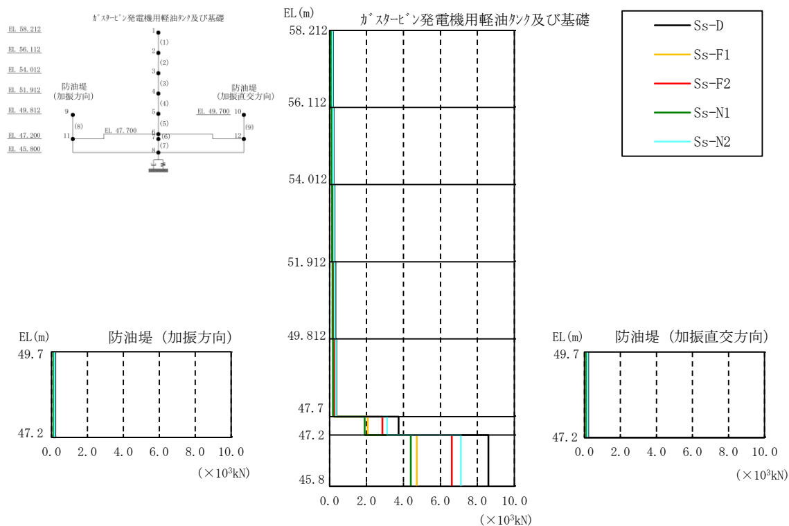
図 3-76 最大応答軸力分布図（解析ケース③）
