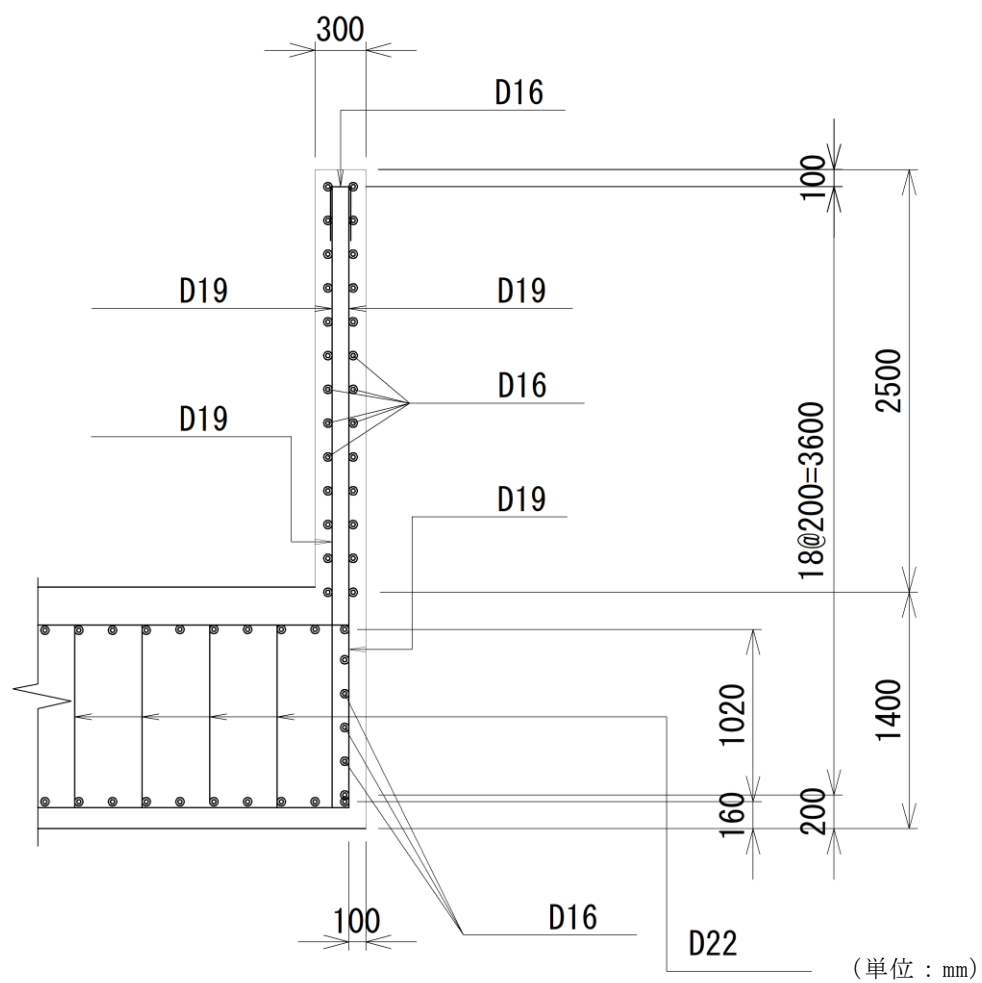
图 3-2 防油堤 概略配筋图 (A-A 断面)
