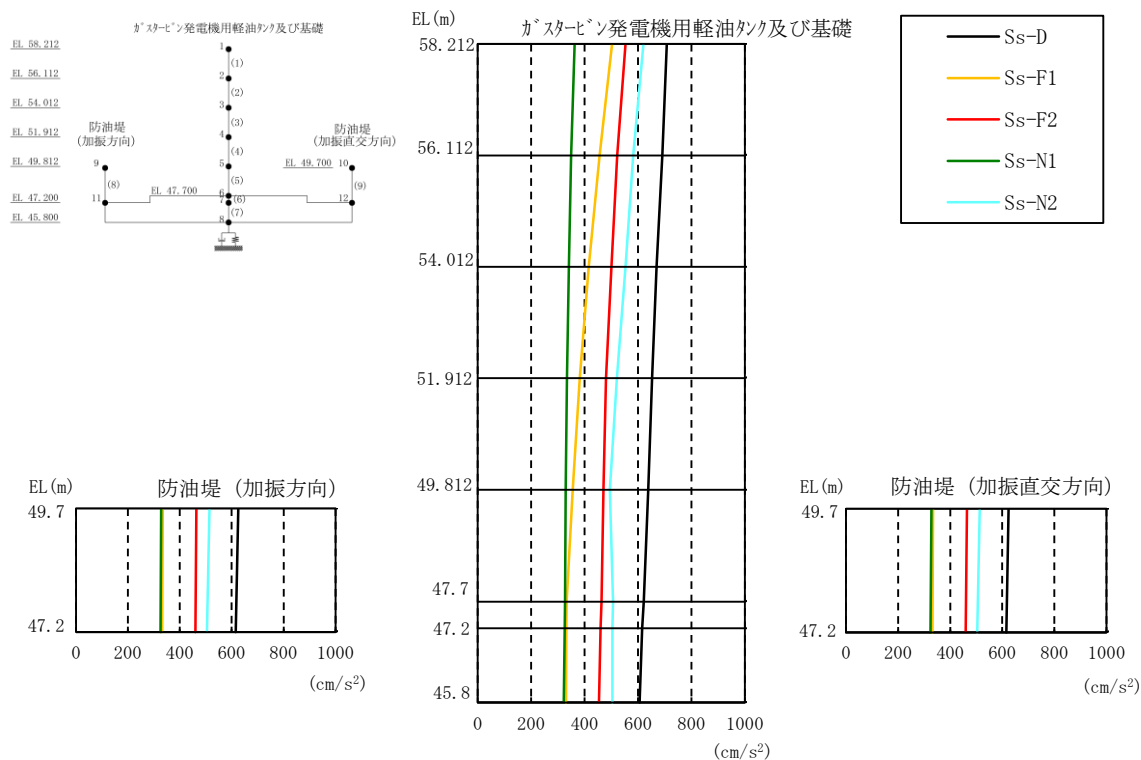
図 3-57 最大応答加速度分布図（鉛直方向，解析ケース①）
