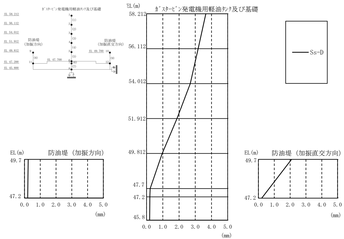
図 1-3 最大応答変位分布図（水平方向，解析ケース④）
