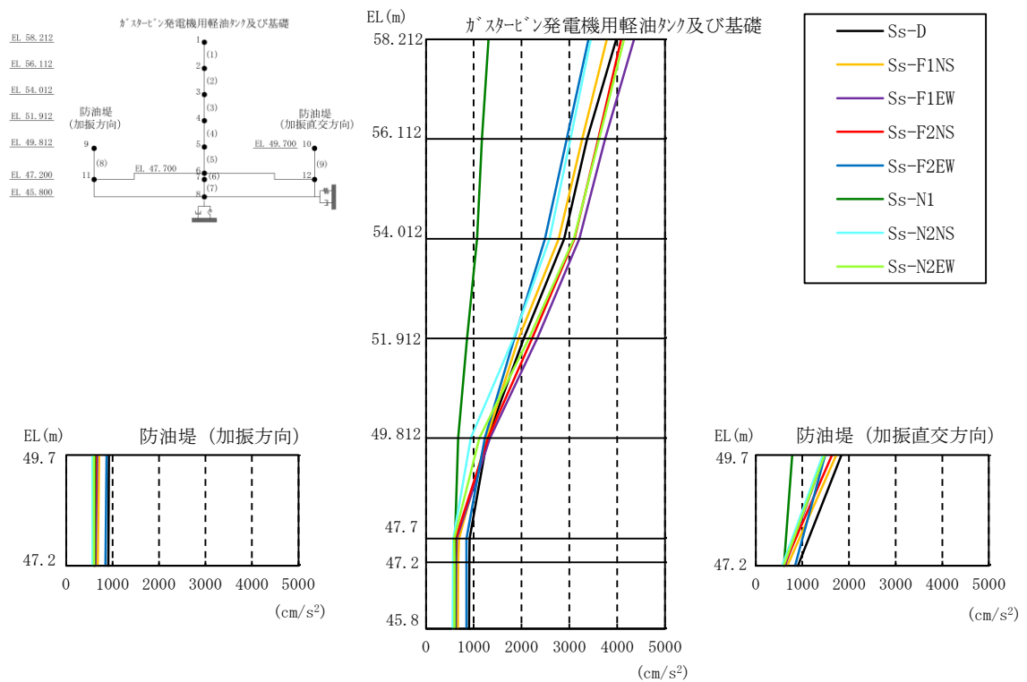
図 3-63 最大応答加速度分布図（水平方向，解析ケース②）
