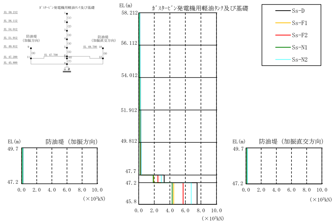
図 3-69 最大応答軸力分布図（解析ケース②）
