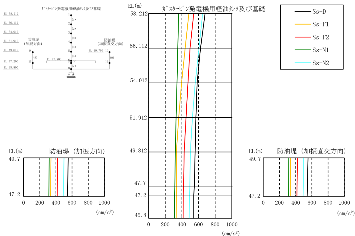
図 3-64 最大応答加速度分布図（鉛直方向，解析ケース②）
