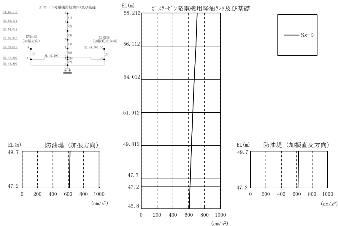
図 1-2 最大応答加速度分布図（鉛直方向，解析ケース④）
