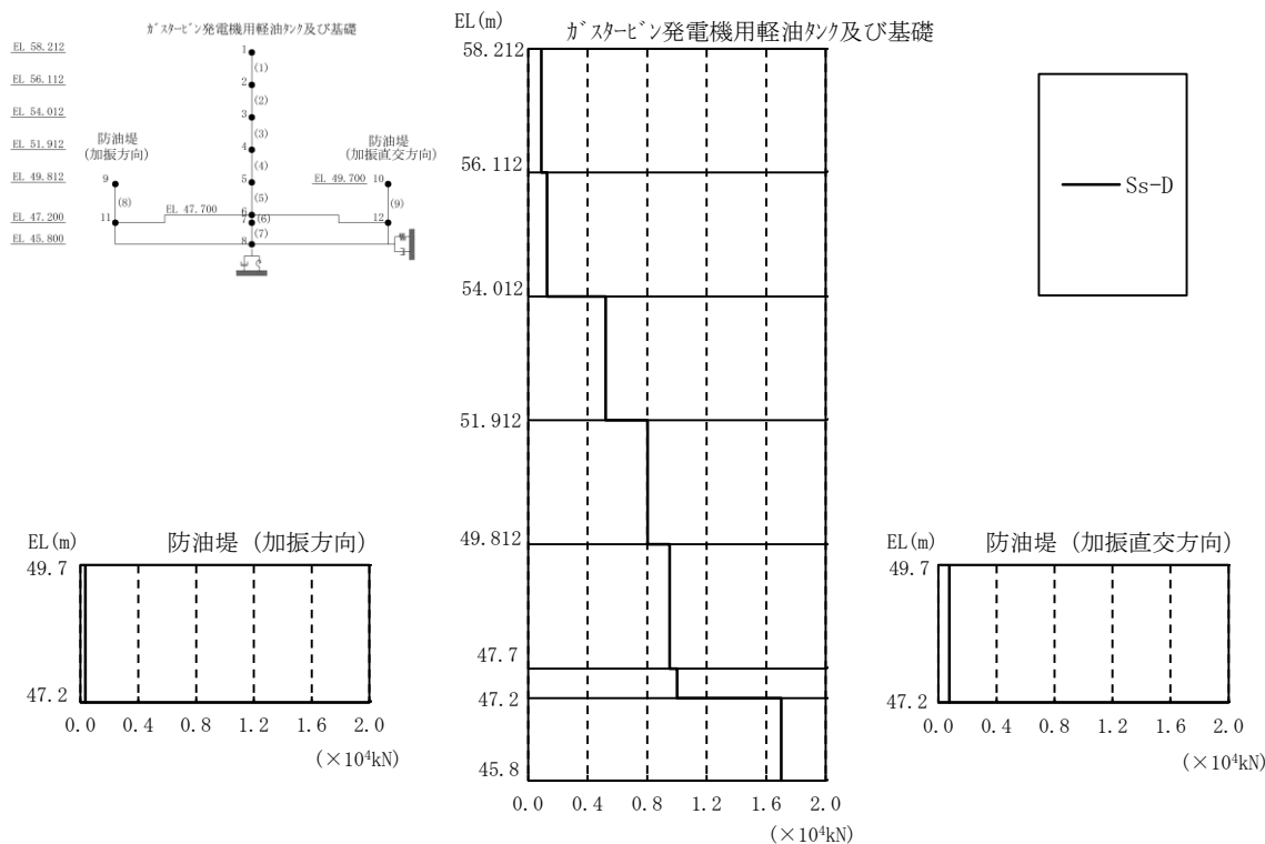
図 1-5 最大応答せん断力分布図（解析ケース④）
