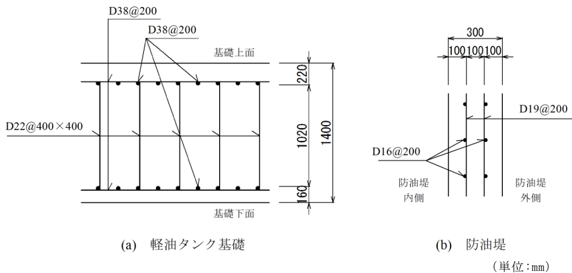
図 2-7 概略配筋図
