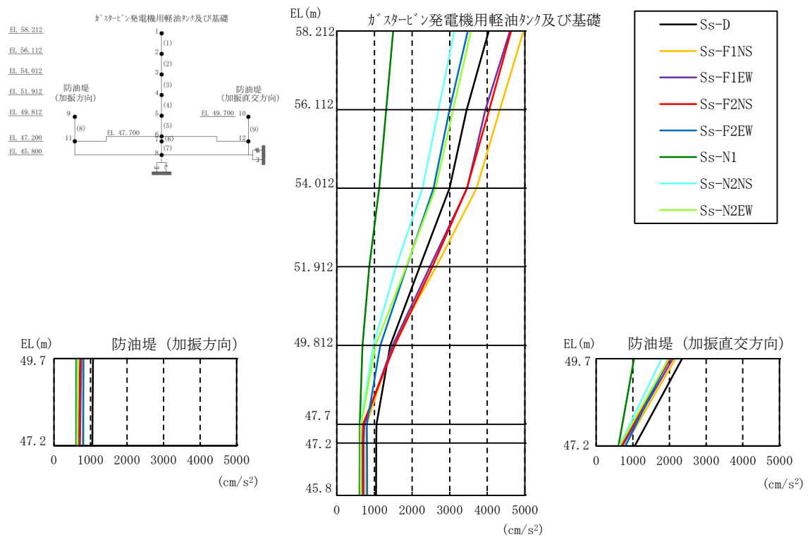
図 3-70 最大応答加速度分布図（水平方向，解析ケース③）
