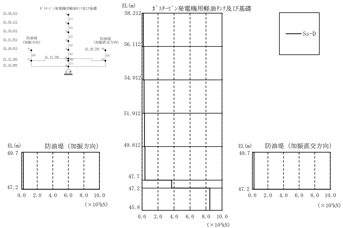
図 1-7 最大応答軸力分布図（解析ケース④）
