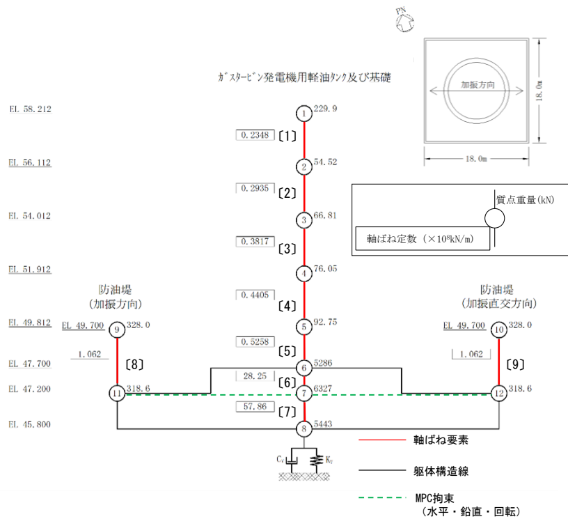
図 3-2 地震応答解析モデル
