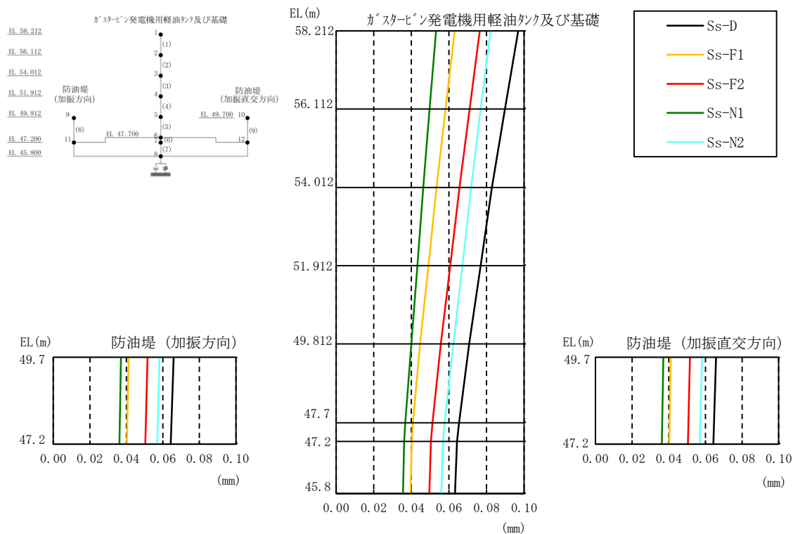
図 3-73 最大応答変位分布図（鉛直方向，解析ケース③）
