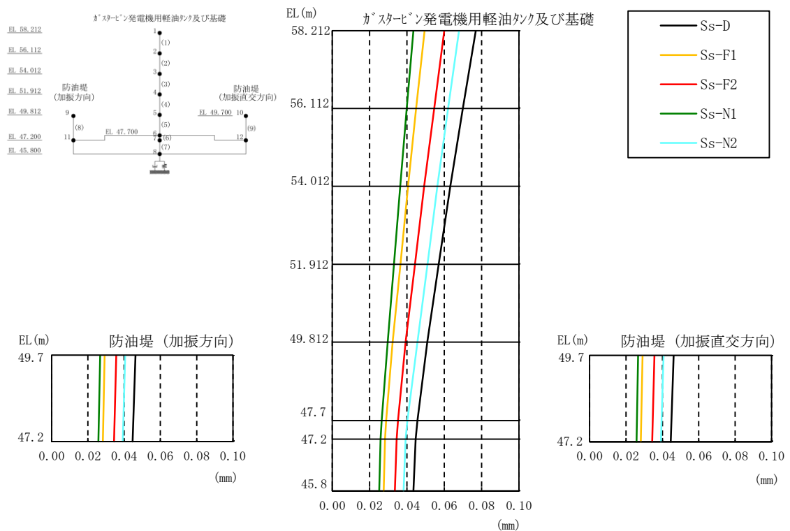
図 3-59 最大応答変位分布図（鉛直方向，解析ケース①）
