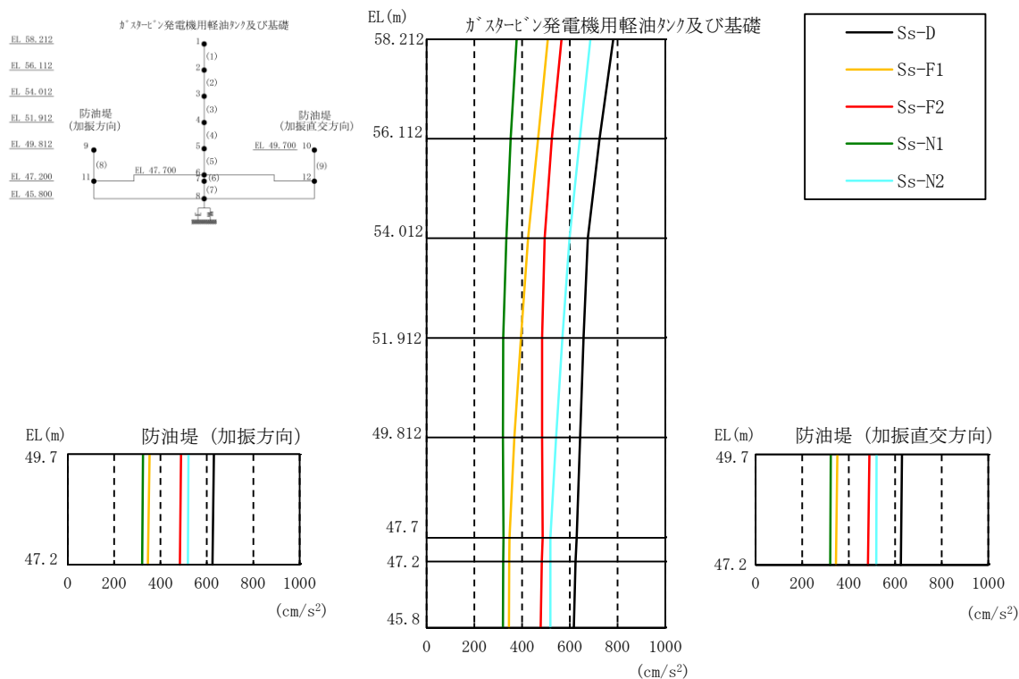
図 3-71 最大応答加速度分布図（鉛直方向，解析ケース③）
