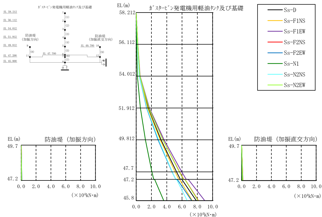
図 3-68 最大応答曲げモーメント分布図（解析ケース②）
