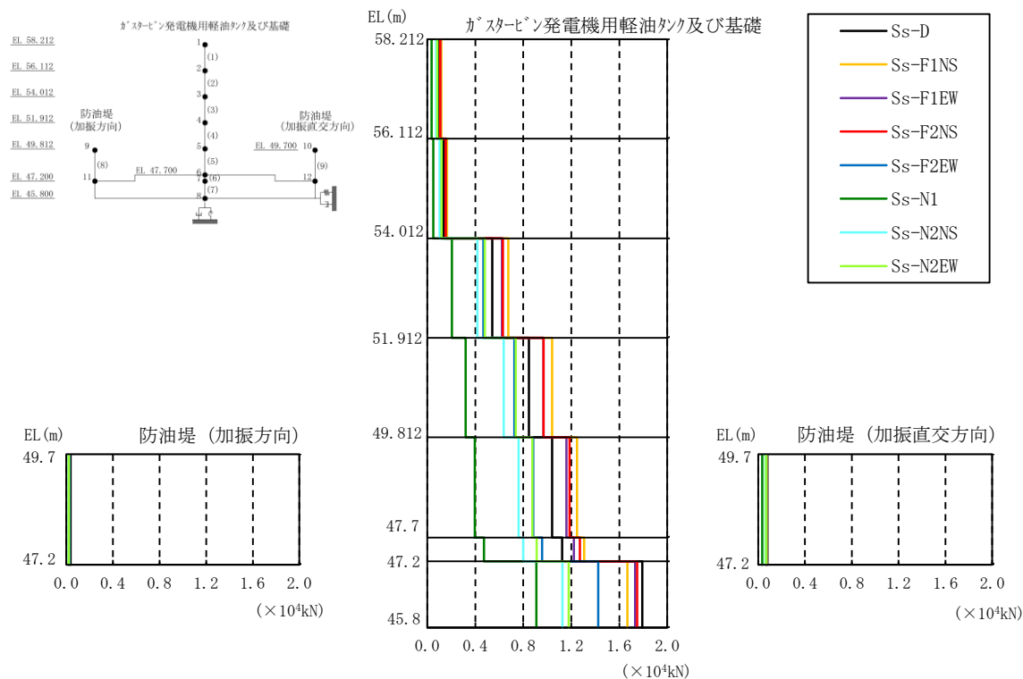
図 3-74 最大応答せん断力分布図（解析ケース③）
