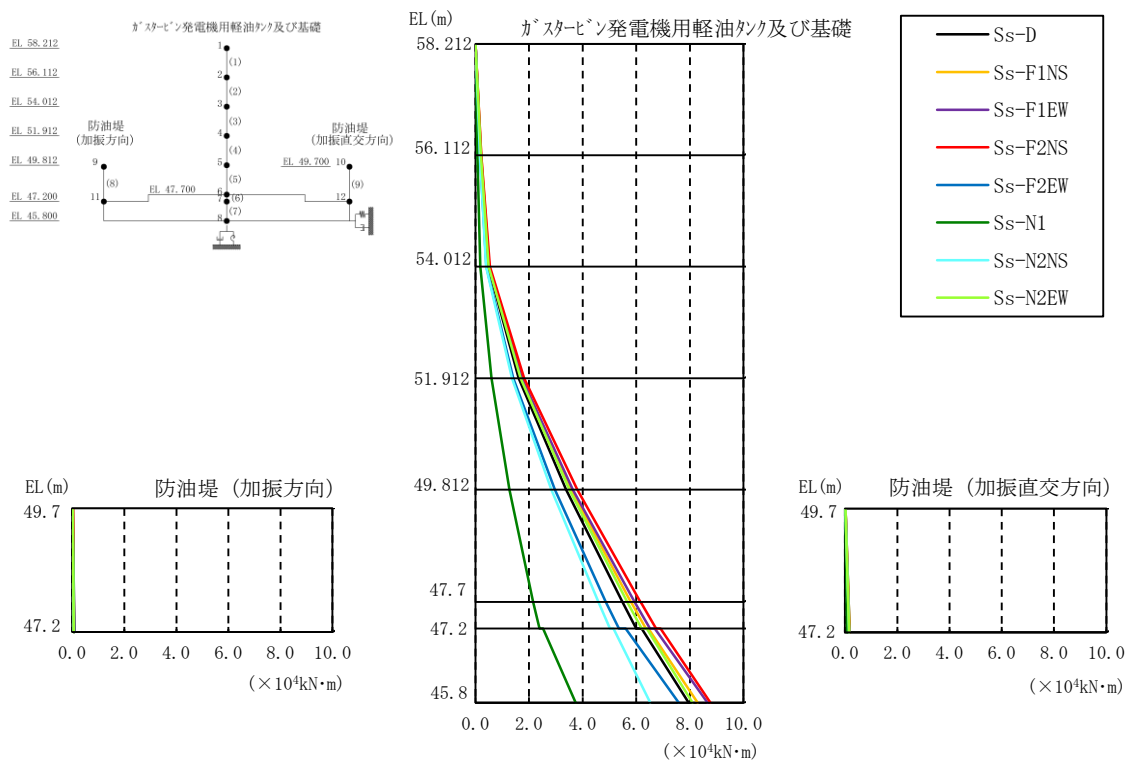
図 3-61 最大応答曲げモーメント分布図（解析ケース①）
