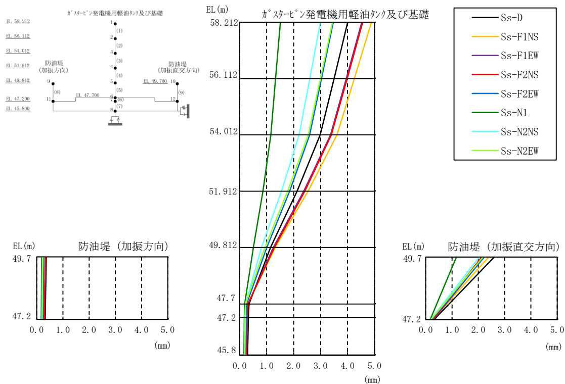
図 3-72 最大応答変位分布図（水平方向，解析ケース③）
