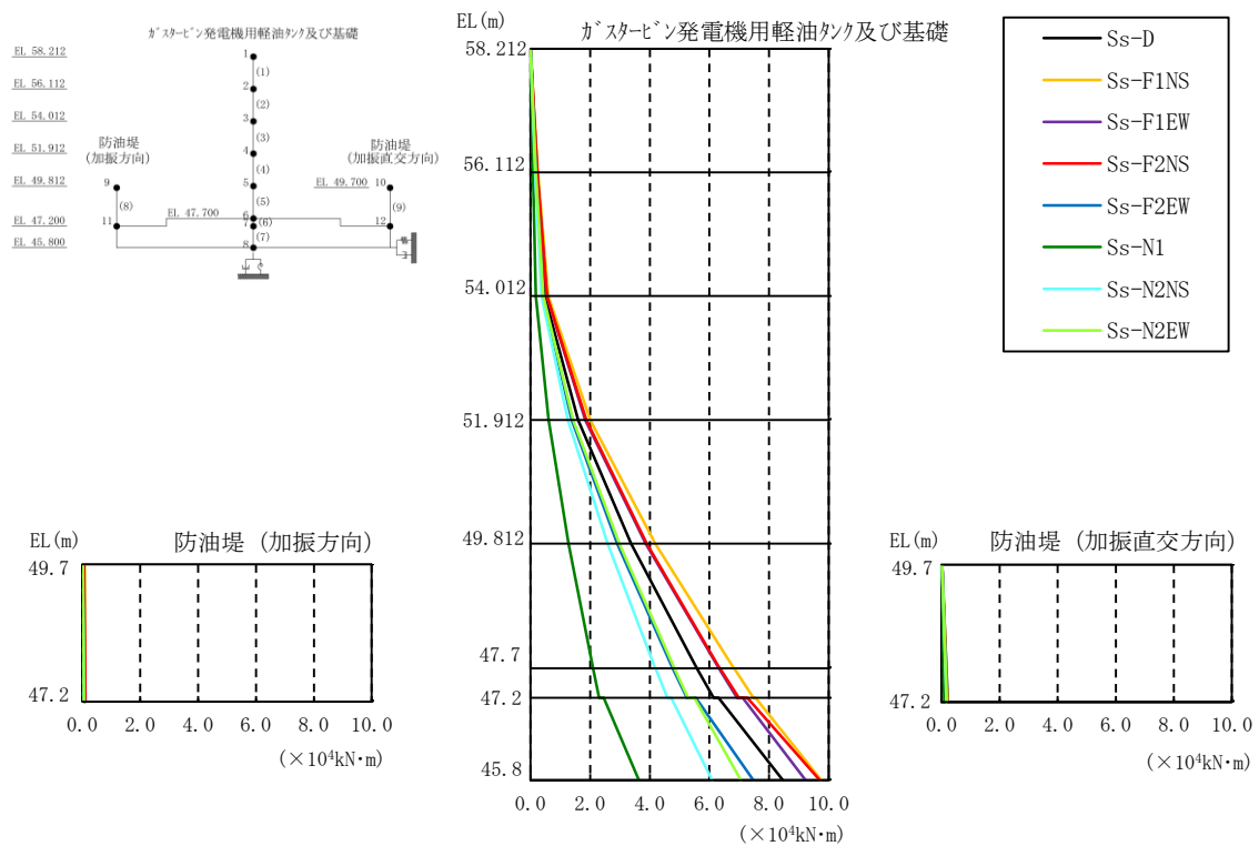
図 3-75 最大応答曲げモーメント分布図（解析ケース③）
