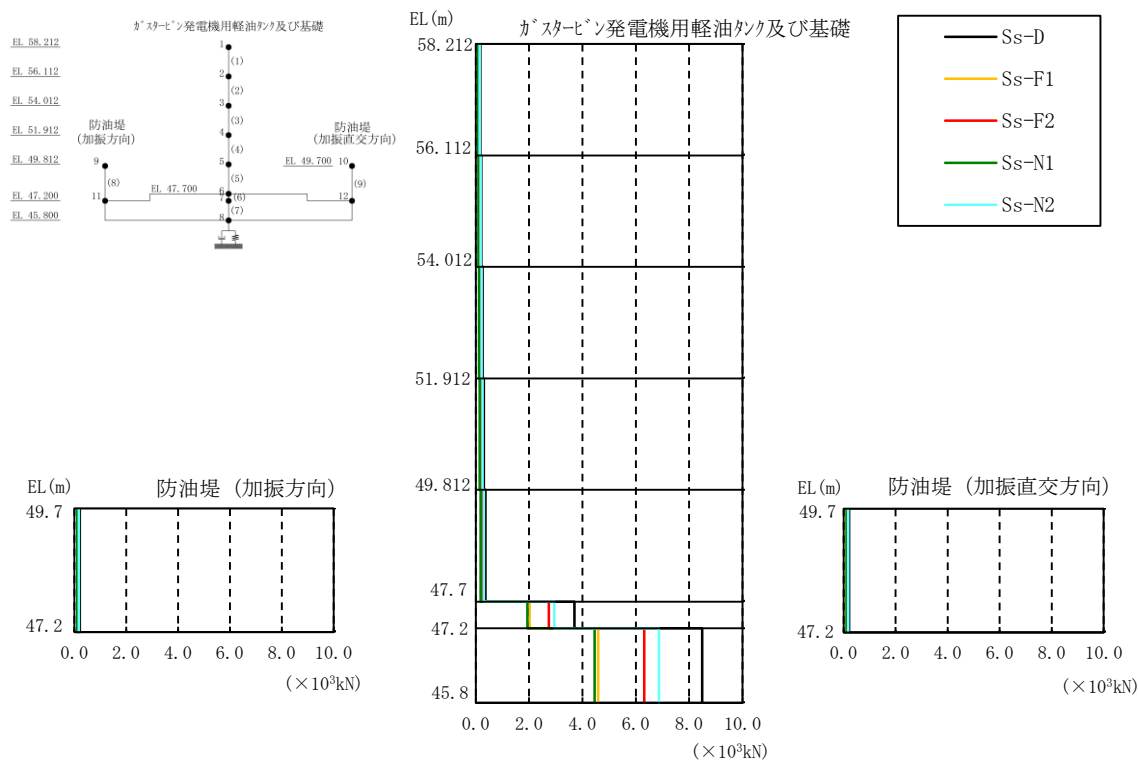
図 3-62 最大応答軸力分布図（解析ケース①）
