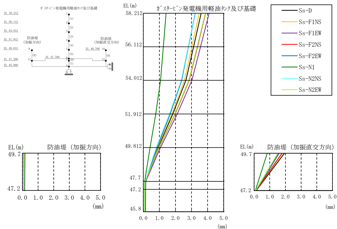
図 3-65 最大応答変位分布図（水平方向，解析ケース②）
