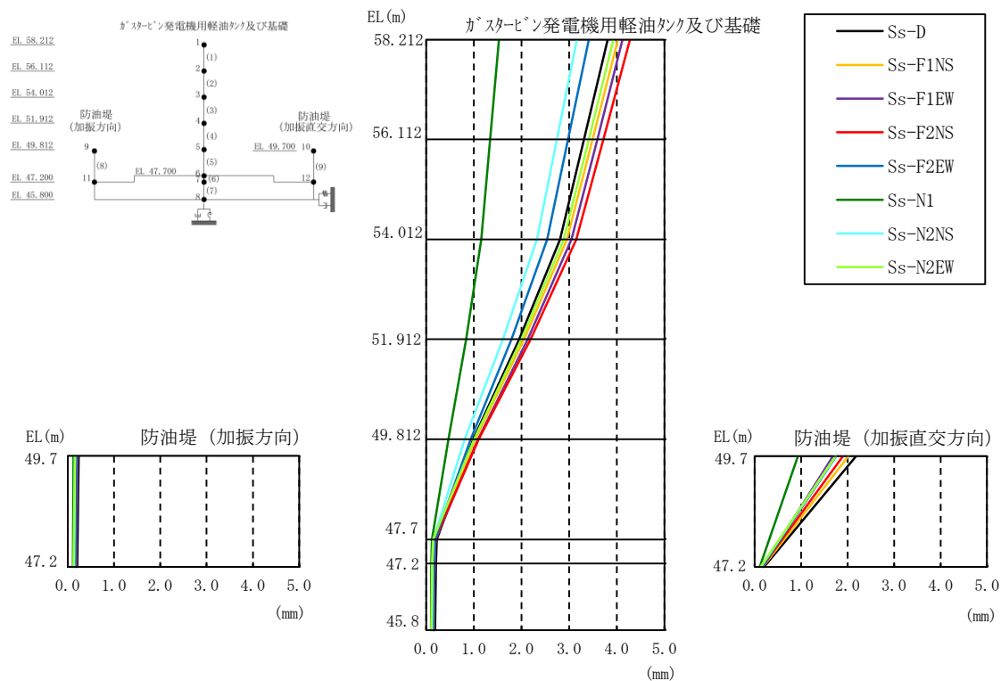
図 3-58 最大応答変位分布図（水平方向，解析ケース①）
