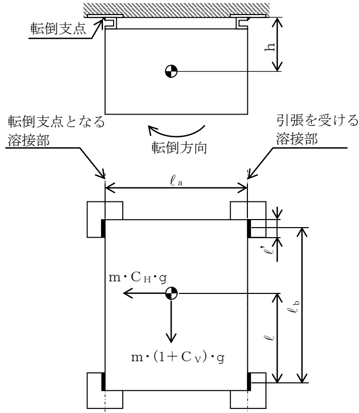
図5-1 計算モデル（溶接部）（左右方向転倒）
