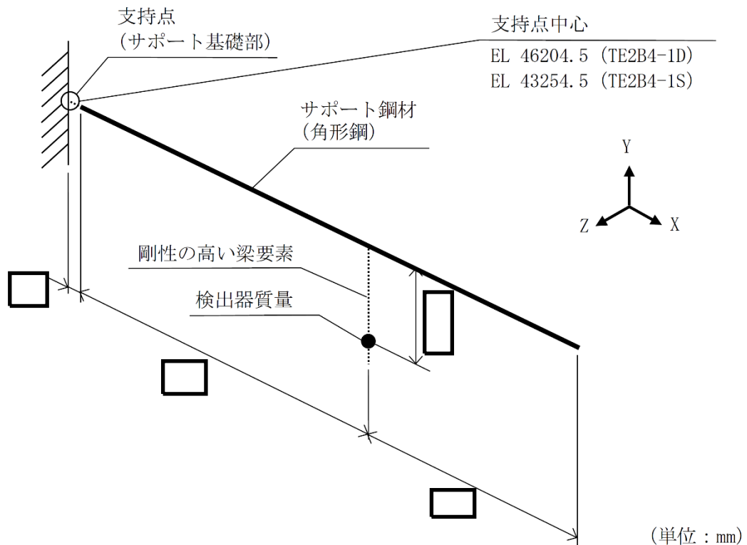
図 4-1 解析モデル
