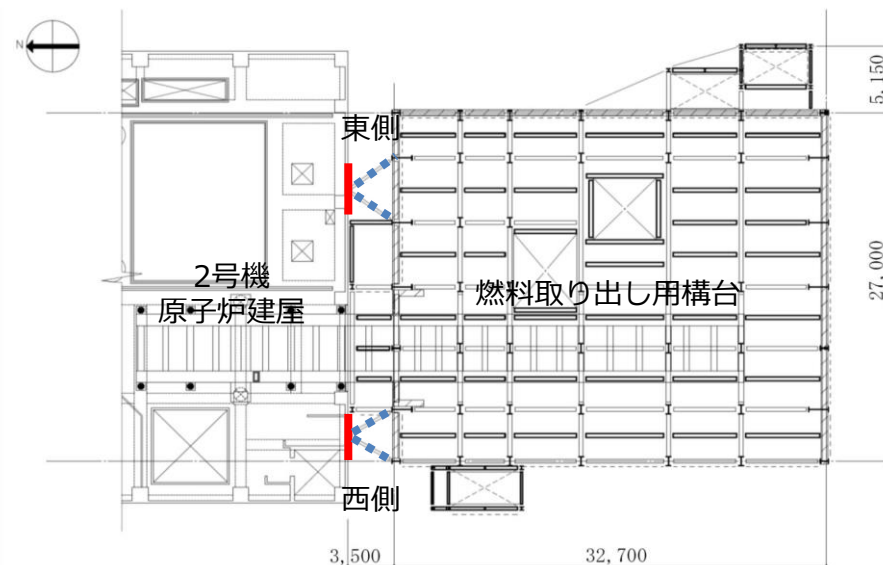
図2 前室床伏図 (G.L.+29,420)
