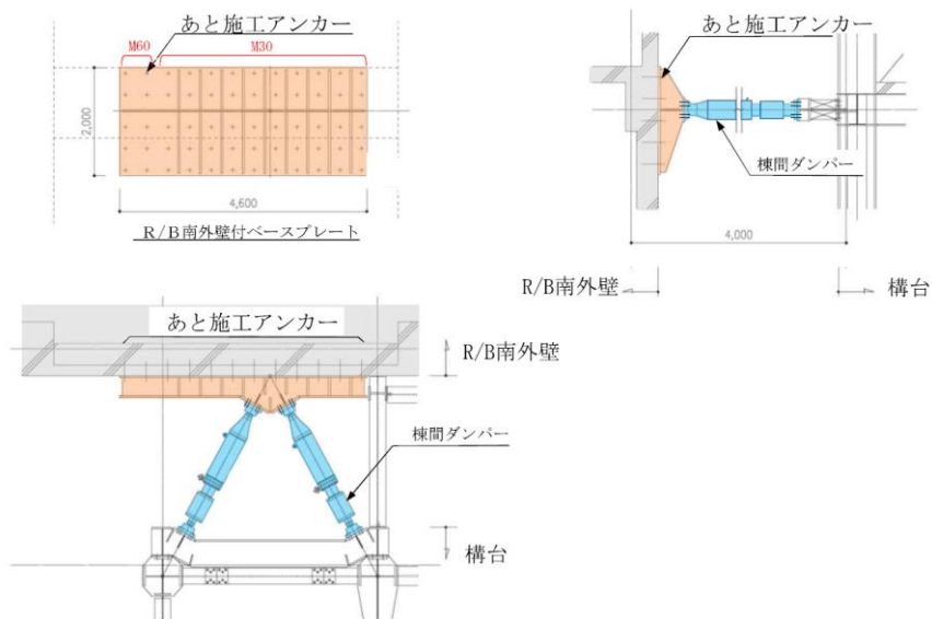
図1 棟間ダンパー接続図
