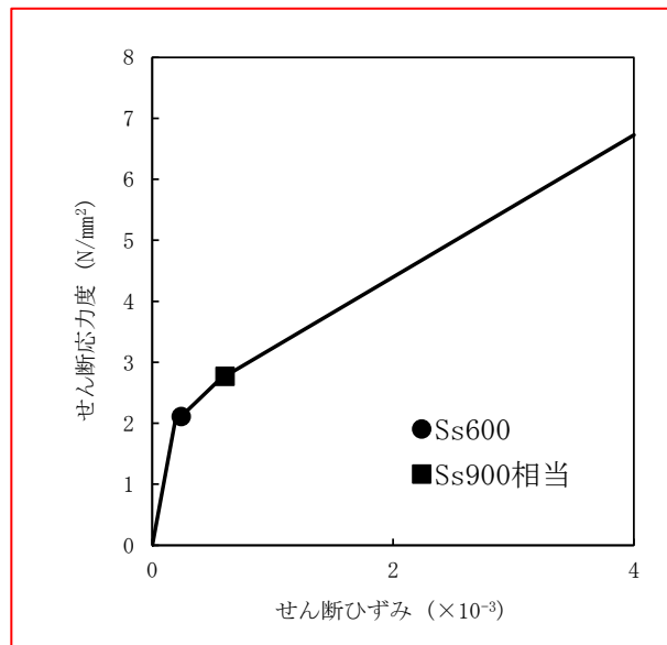
図1 せん断スケルトン曲線上の最大応答値
