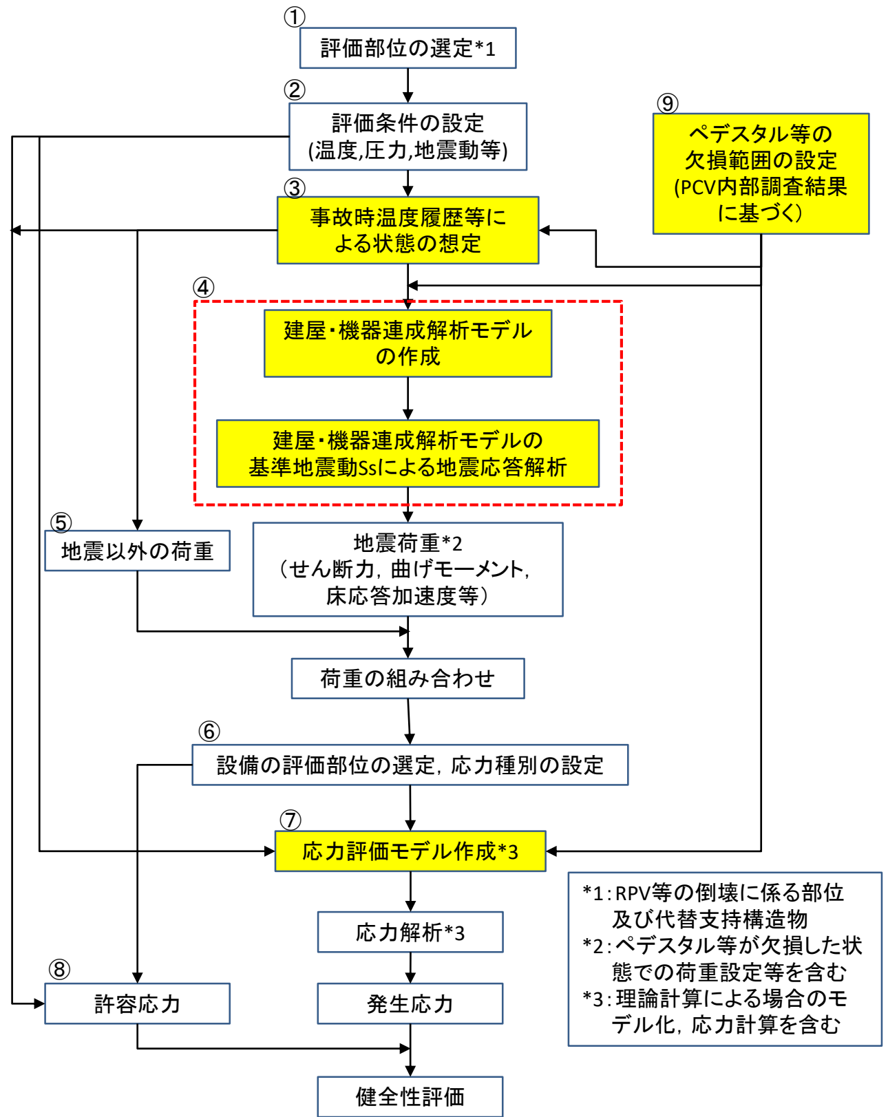
図1. 健全性評価フロー
