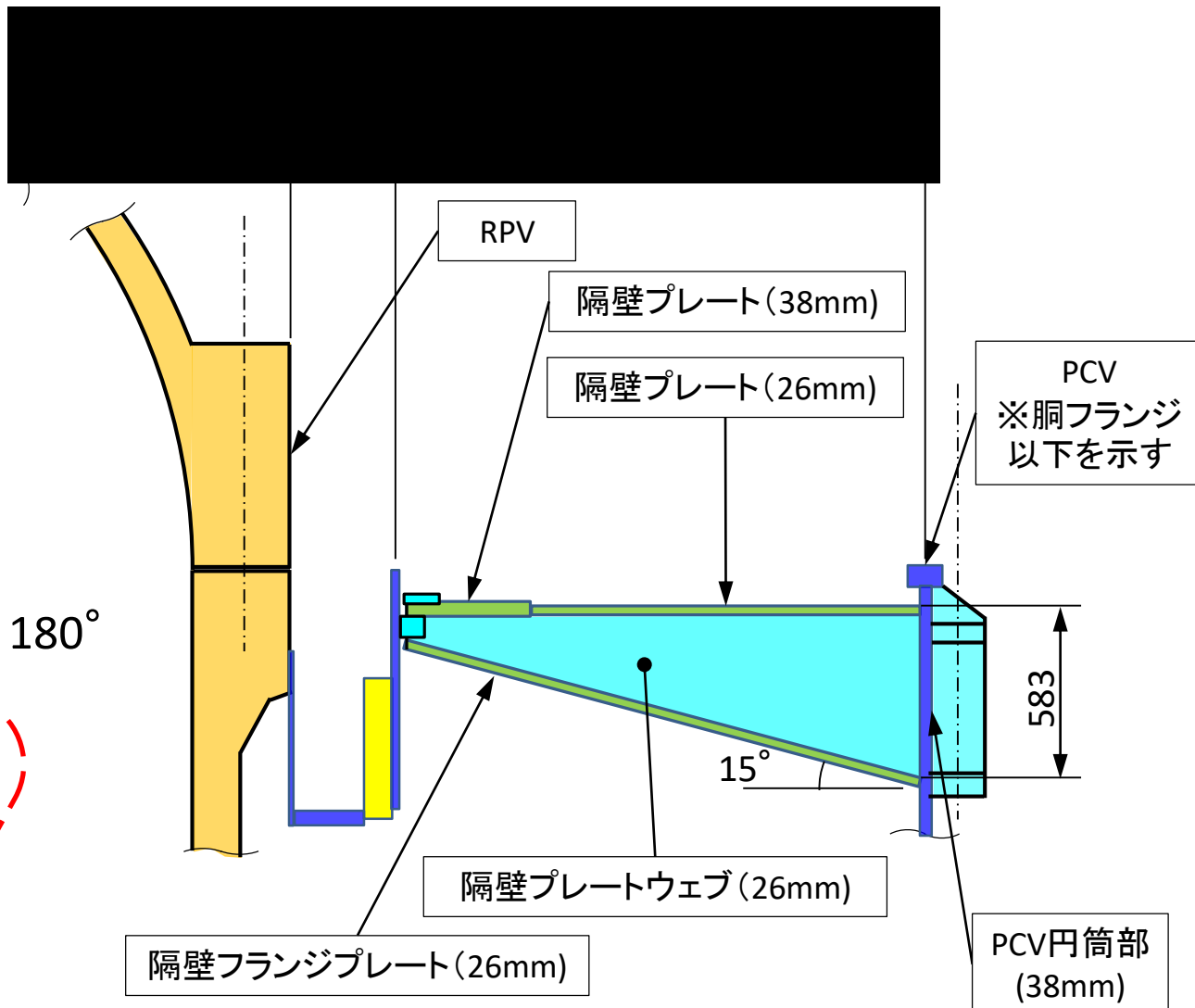
図.3- 2 バルクヘッドの断面概要
