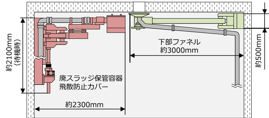
A-A矢視図
