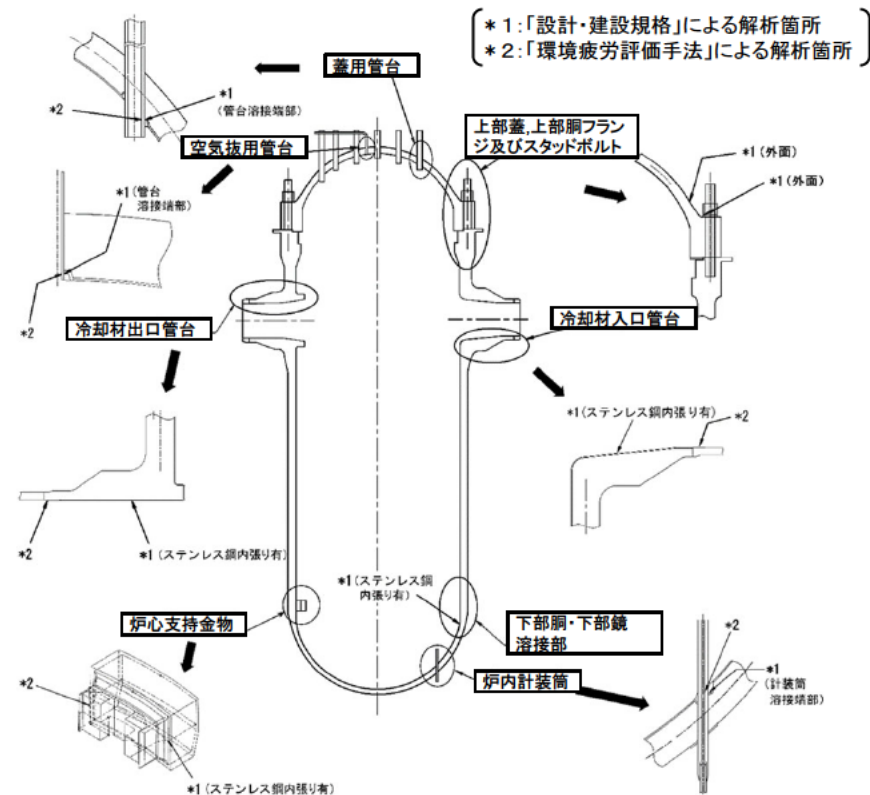
図 原子炉容器の疲労評価対象部位
