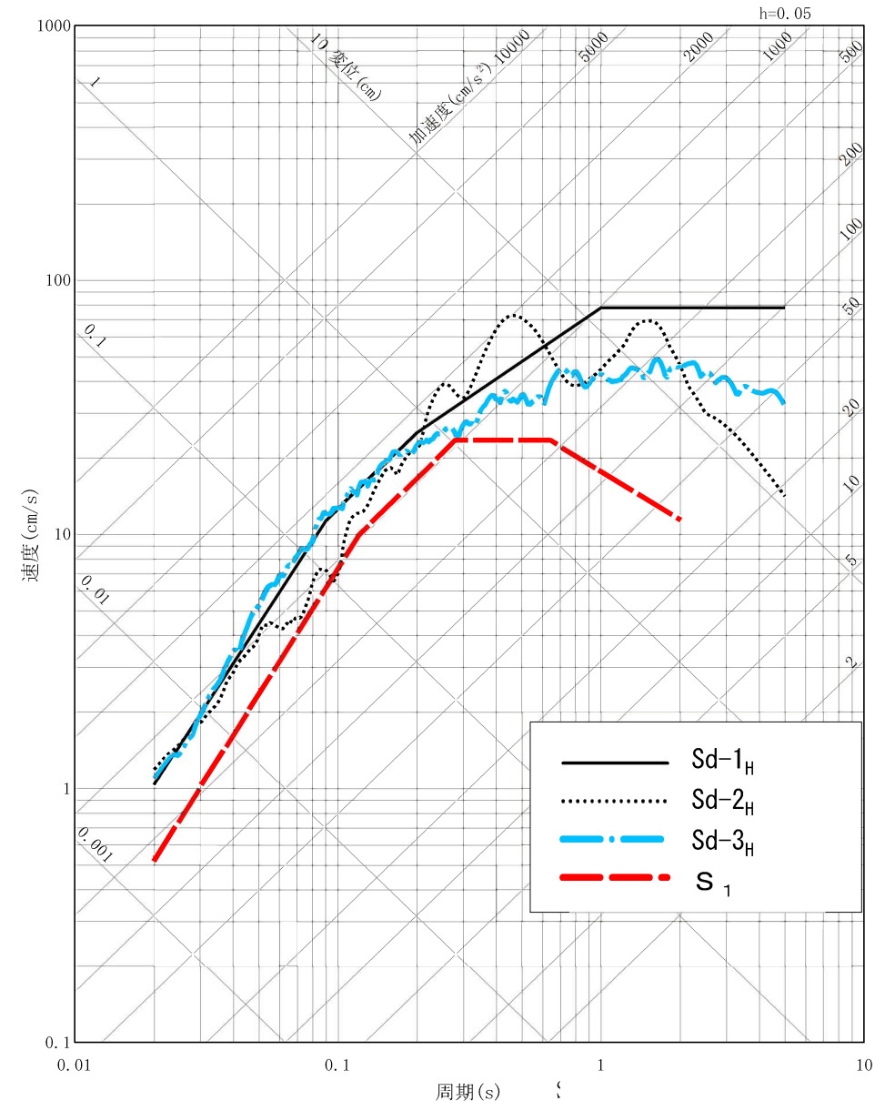
弾性設計用地震動Sd-3と基準地震動S 1 の 応答スペクトルの比較
