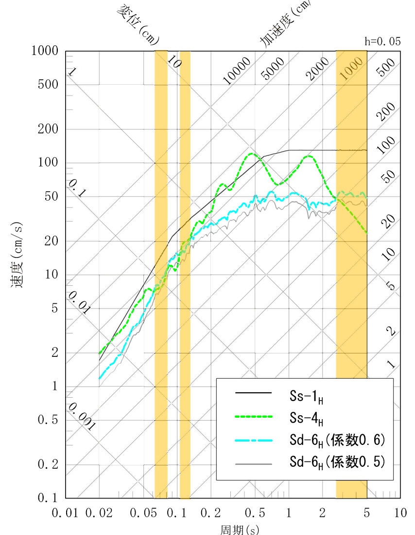
※黄ハッチング箇所はSd-6 H (係数0.6) > Ss-4 H となる周期帯を示す
