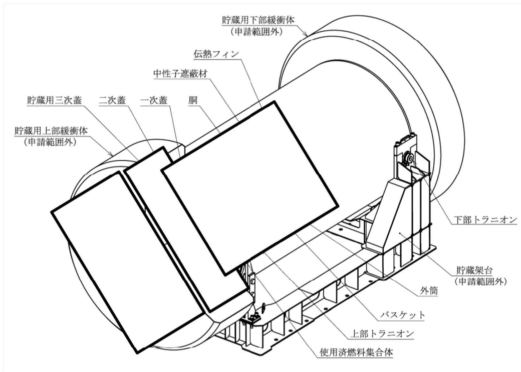
[実形状] 三次元モデル化
