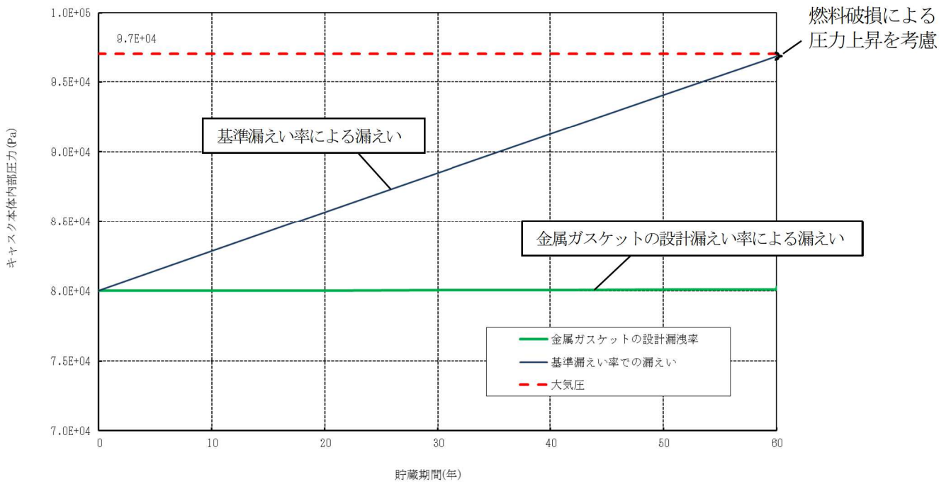
第5図 特定兼用キャスク内部圧力の経時変化
