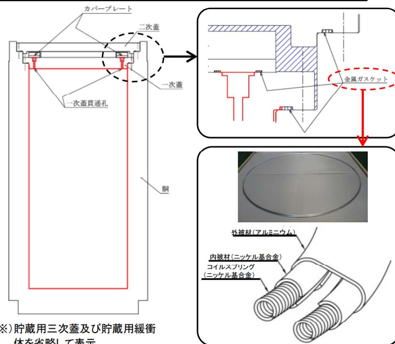
閉じ込め構造図
