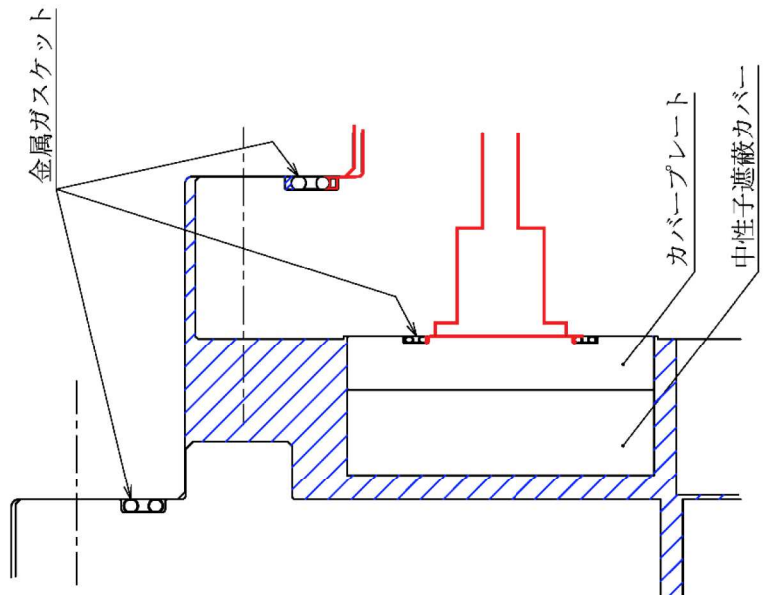
A部詳細
