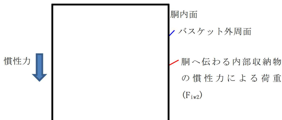
別添 2 - 3 - 2 図 MSF-28P 型の胴内面とバスケット外周面の形状
