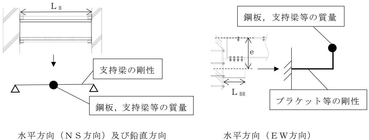
図 4-1 固有周期の計算モデル
