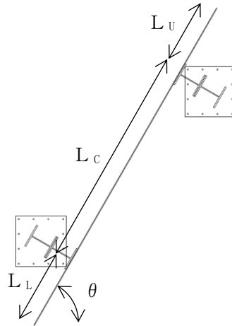
図5-1 鋼板の計算モデル図
