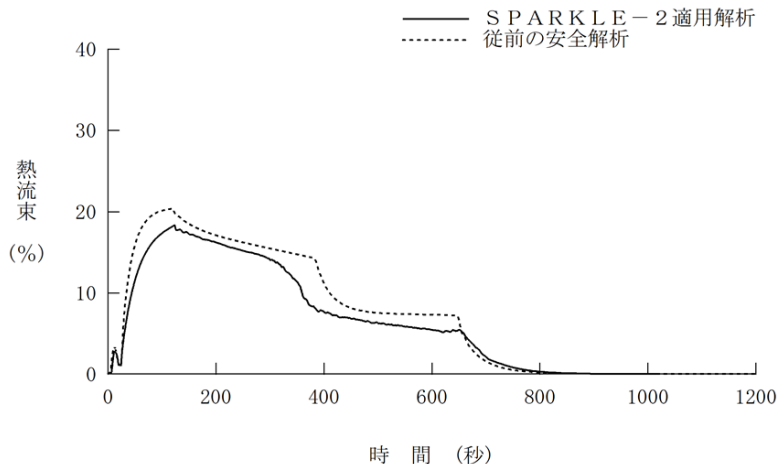
「主蒸気管破断」解析結果（熱流束）
