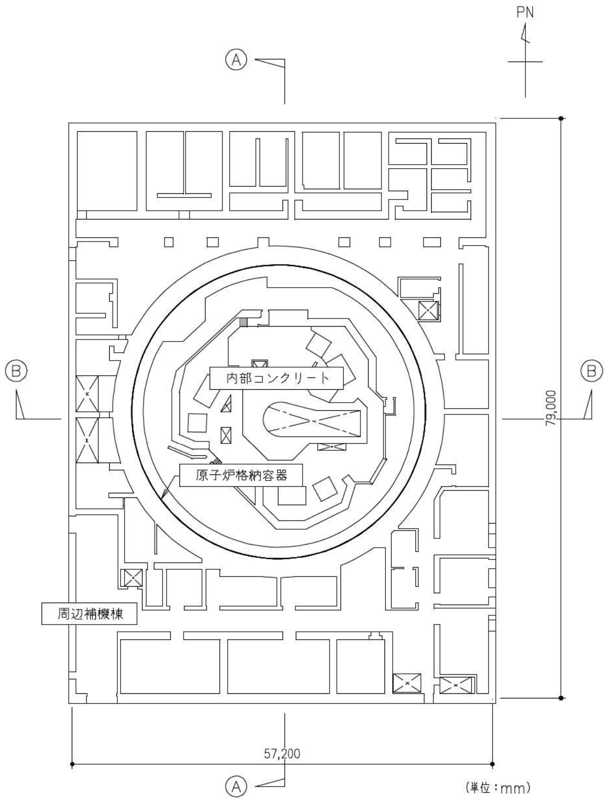
第 8-2 図(1) 原子炉建屋の概略平面図 (T. P. 10.3m)
