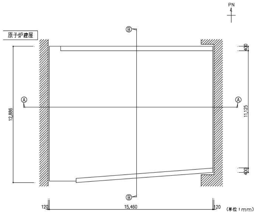
第 8-33 図 原子炉建屋栈橋の概略平面図
