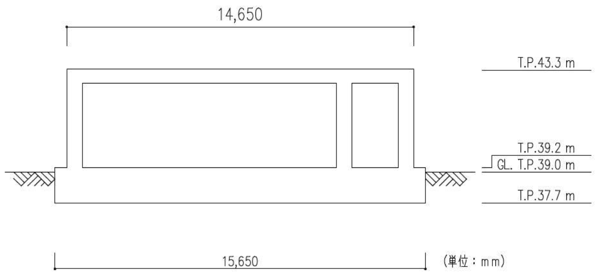
第 8-15 図(2) 空調上屋の概略断面図 (B-B断面)
