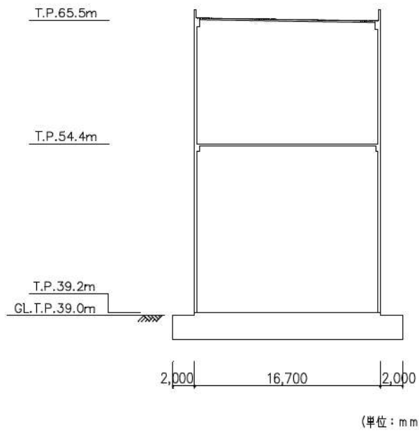
第 8-23 図(2) 定検機材倉庫の概略断面図 (B-B断面)
