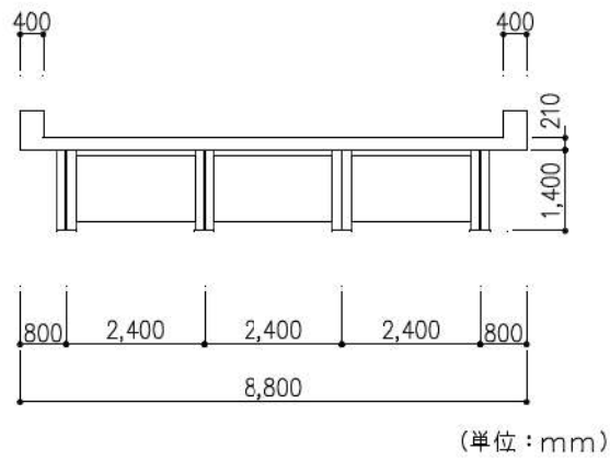
第 8-38 図(2) 原子炉補助建屋棧橋の概略断面図 (B-B断面)
