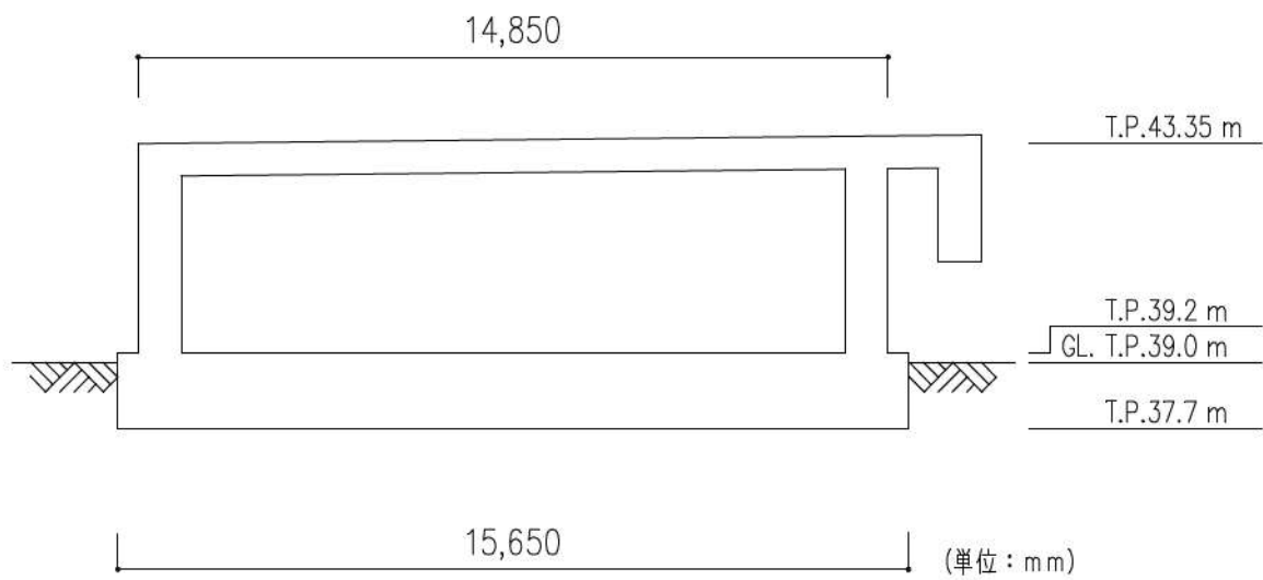
第 8-13 図(1) 緊急時対策所の概略断面図 (A-A断面)
