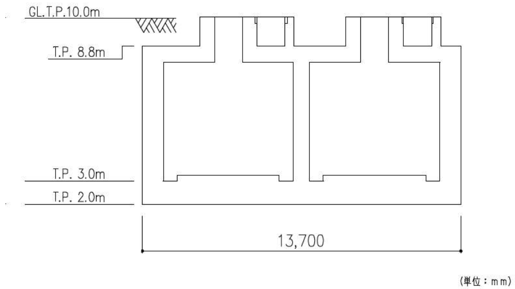
第 8-11 図(1) B1, B2—燃料油貯油槽タンク室の概略断面図 (A—A断面)
