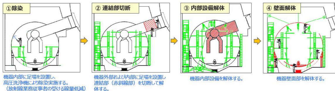
図1 サプレッション・チェンバの解体撤去イメージ
