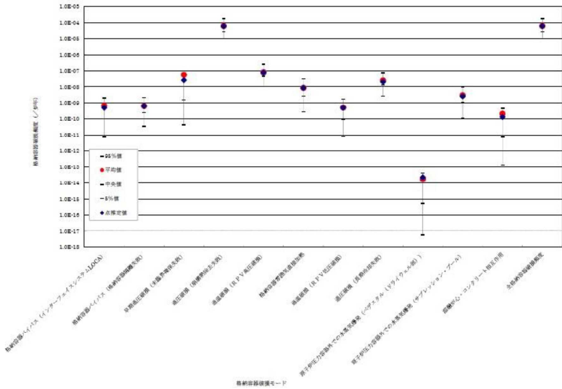
図 1-1 内の事象レベル 1.5PRA 評価結果 (Mark-I 改)
