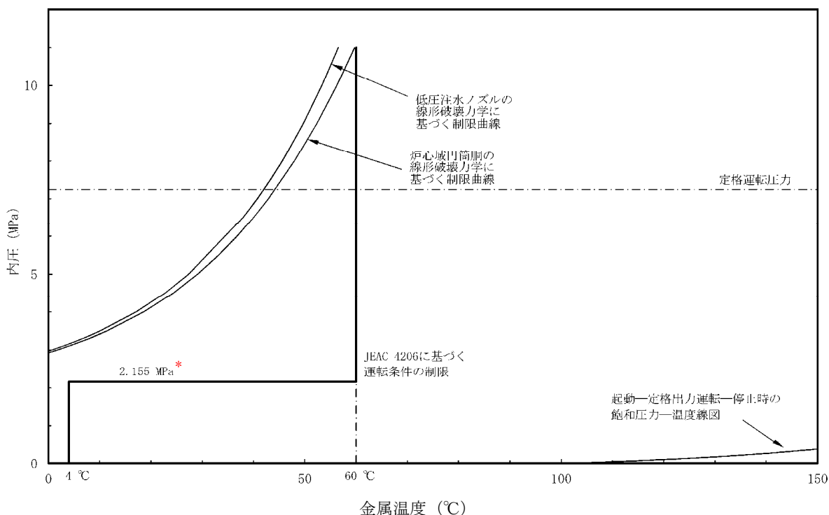
図 8 原子炉圧力容器の圧力－温度制限線図（運転開始後 60 年時点，炉心臨界時）(1/2)
