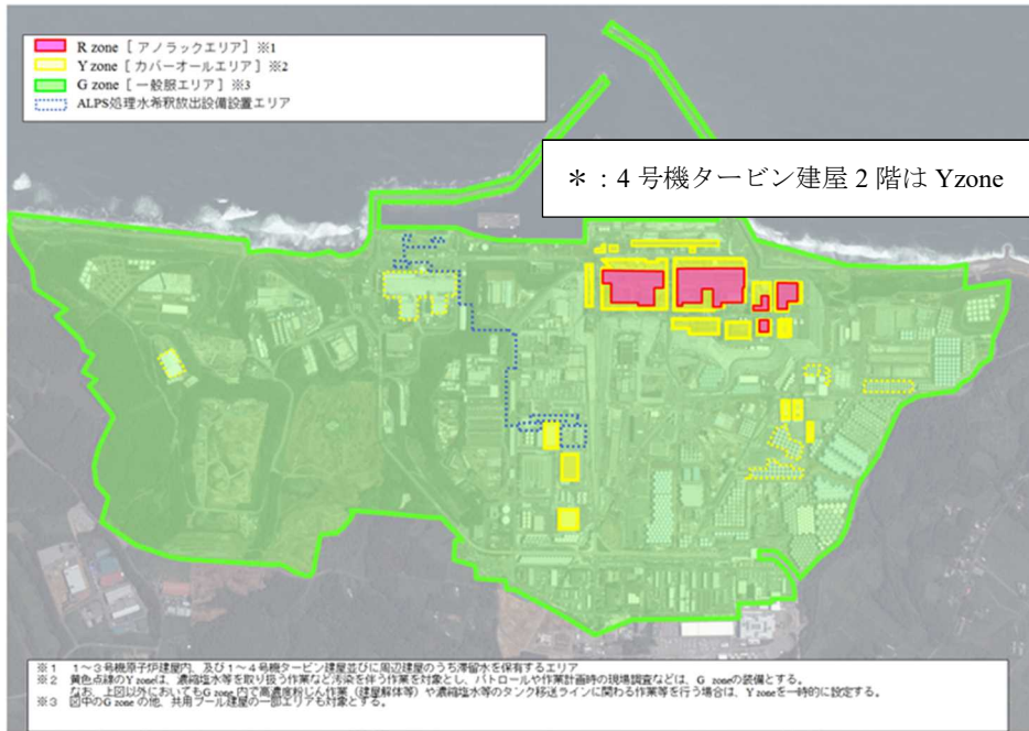
図 2.12.1-2 建屋内RO処理水移送配管設置工事の作業エリアの区域区分図
