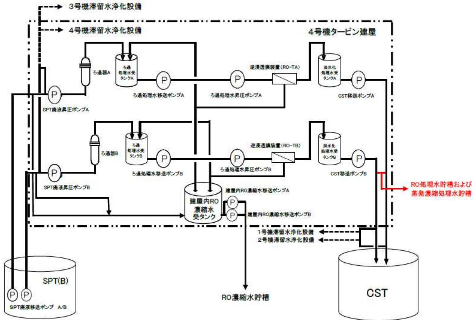
図2.14.1-1 淡水化装置（逆浸透膜装置，蒸発濃縮装置）及び滞留水浄化設備の系統構成図（2/2） （滞留水浄化設備の範囲について点線で示す。）
