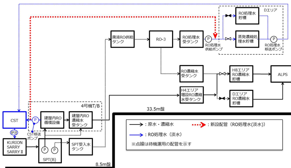
図 1.1-1 系統概略図
