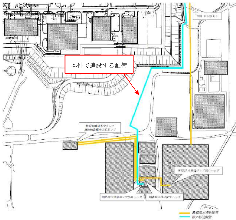
図 1.1-2 配置概略図 (2 / 2)
