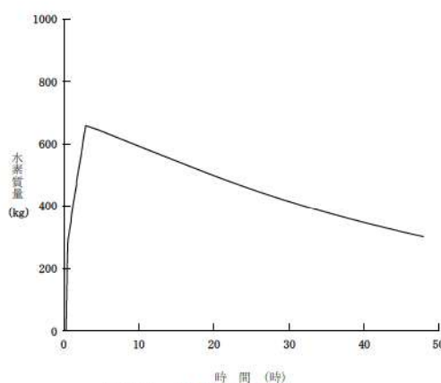
図 29 発生水素量
