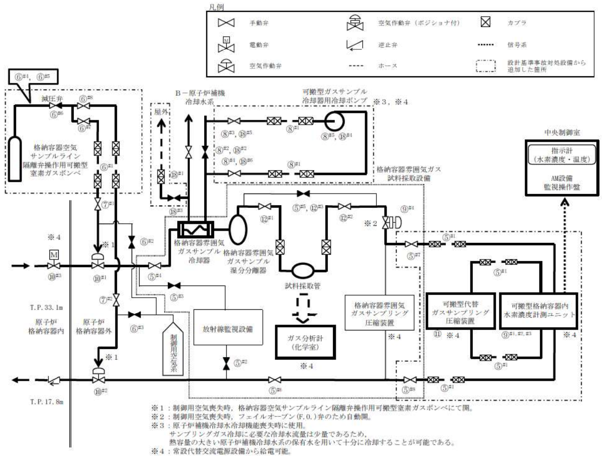
第 1.9.10 図 ガス分析計による原子炉格納容器内の水素濃度監視（全交流動力電源及び原子炉補機冷却機能が喪失した場合） 概要図（1/3）
