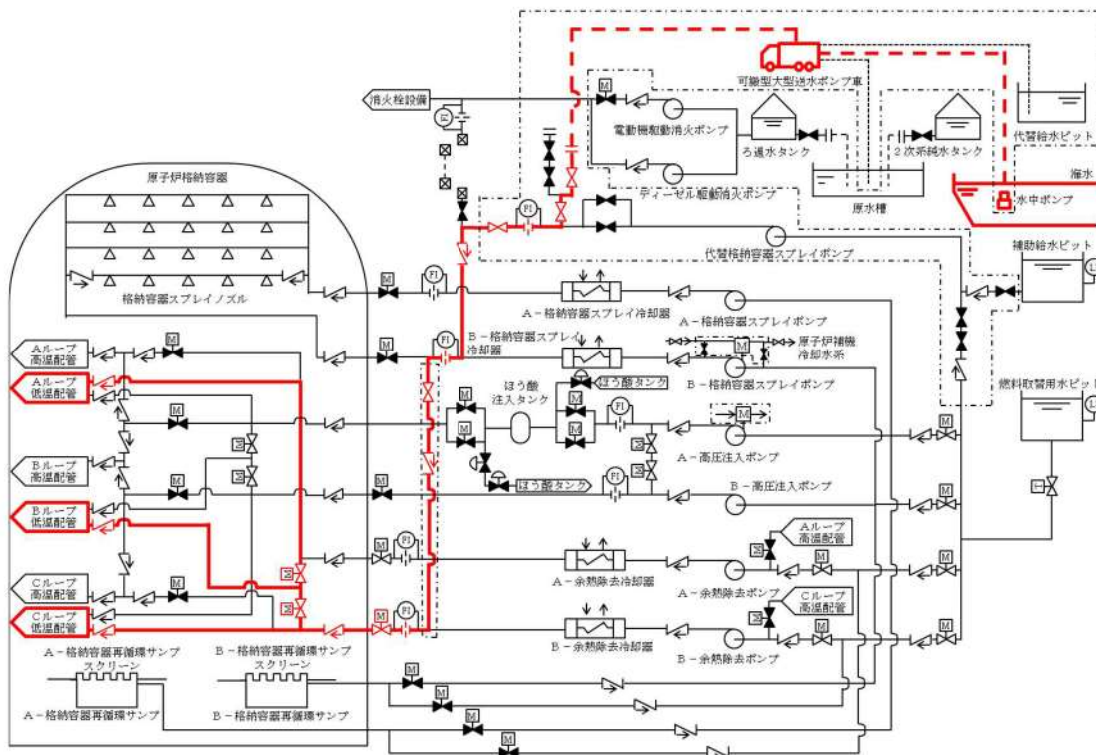
代替炉心注水（可搬型大型送水ポンプ車）
