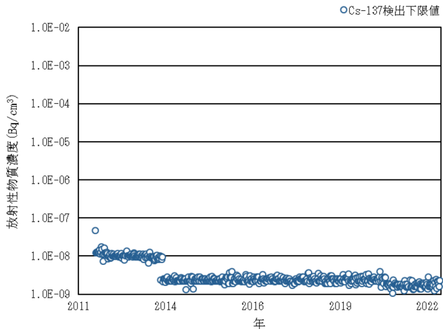
図 A. 4-22-11-3 5, 6 号機共用排気筒からの粒子状物質放出濃度推移 (実施計画：III-3-2-1-3-9)
