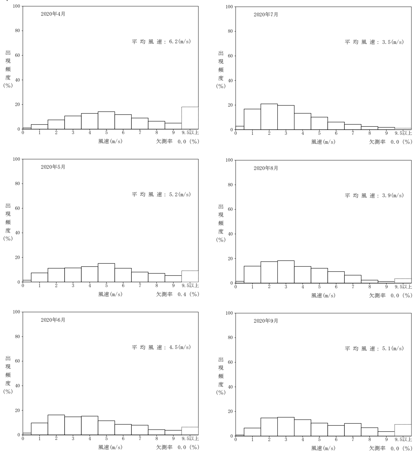
図 A. 2-14 月別風速別出現頻度(その 3) (2020 年 4 月～2020 年 9 月)
