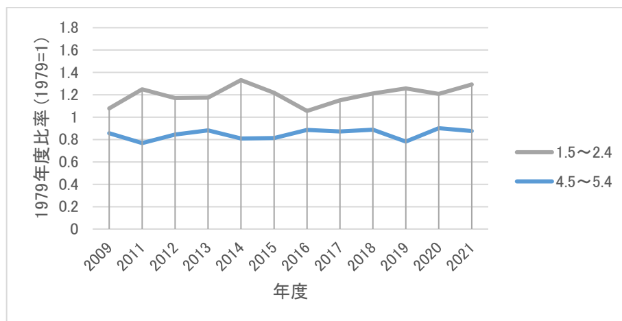
図 A.1-2 風速分布出現頻度の経年変化
