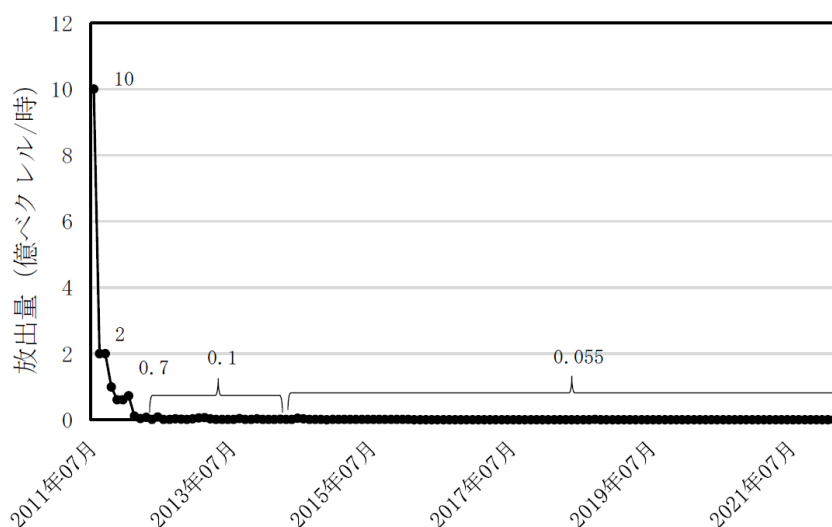
図A.4-12.11-22 1～4号機原子炉建屋からの一時間当たりの放出量推移 (実施計画：III-3-2-1-3-8)
