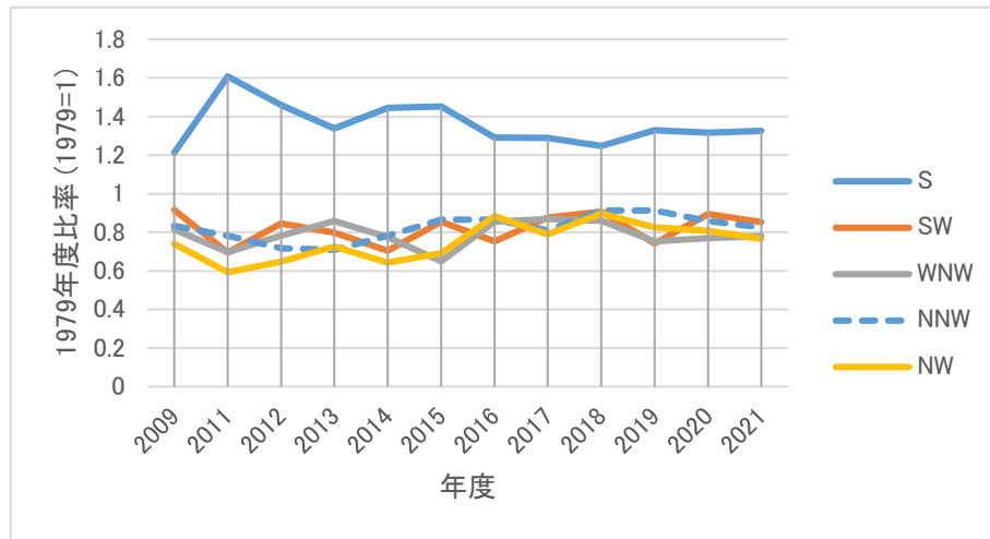
図 A.1-1 風向頻度の経年変化
