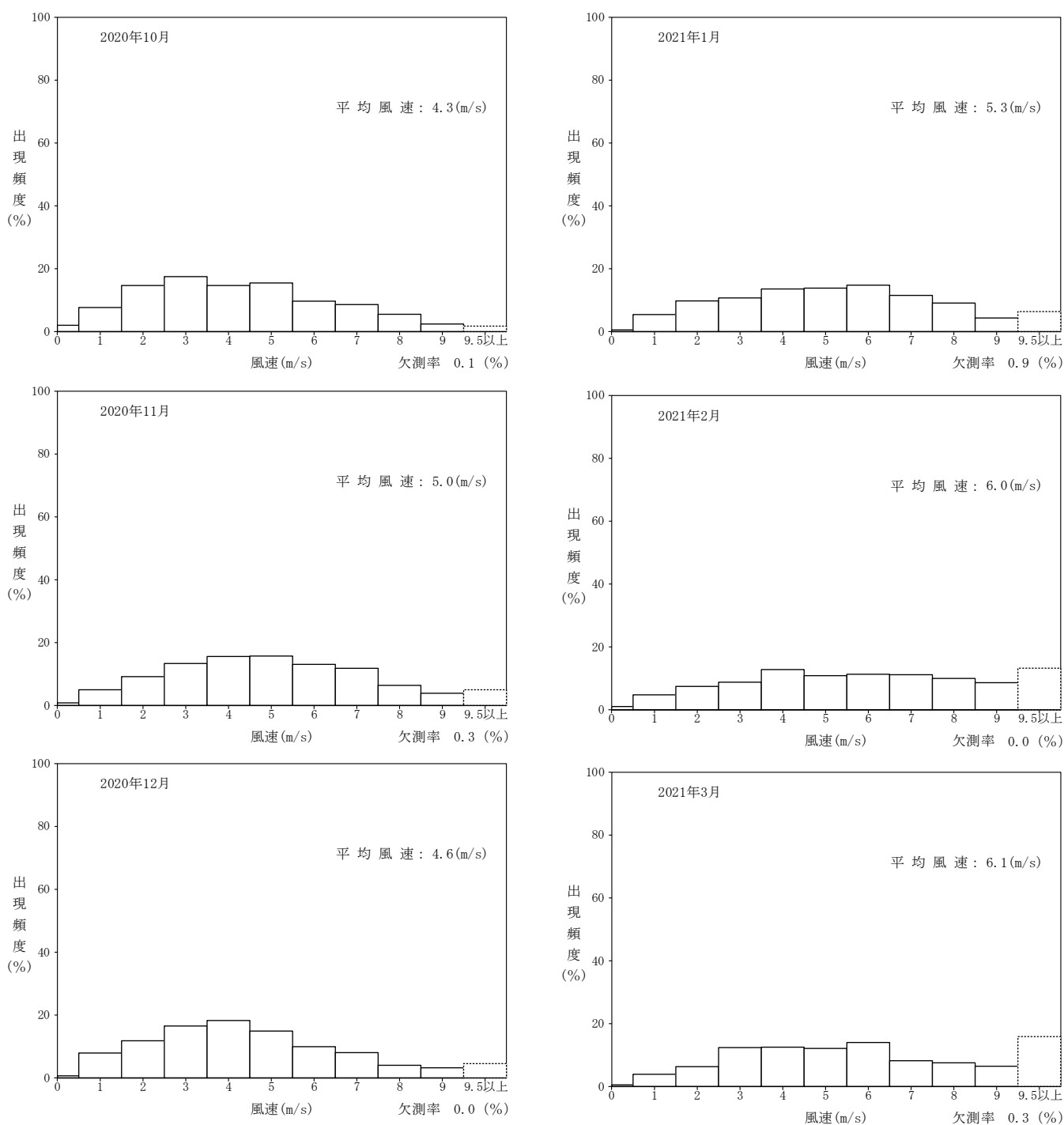
図 A. 2-15 月別風速別出現頻度(その4) (2020年10月～2021年3月)
