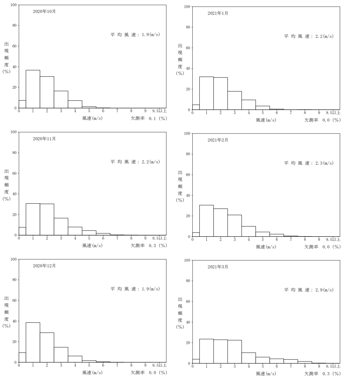
図 A. 2-13 月別風速出現頻度 (その2) (2020年10月~2021年3月)
