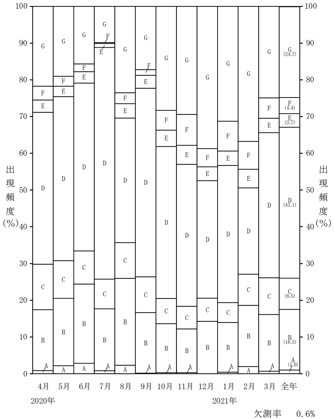
図 A. 2-16 年間及び月別大気安定度出現頻度
