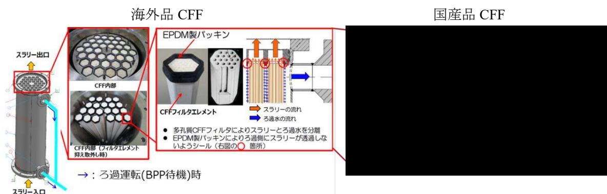
図 2.14.1-1 CFF 構造について
