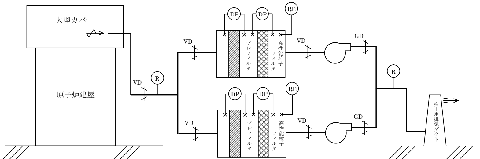
大型カバー換気設備系統図
