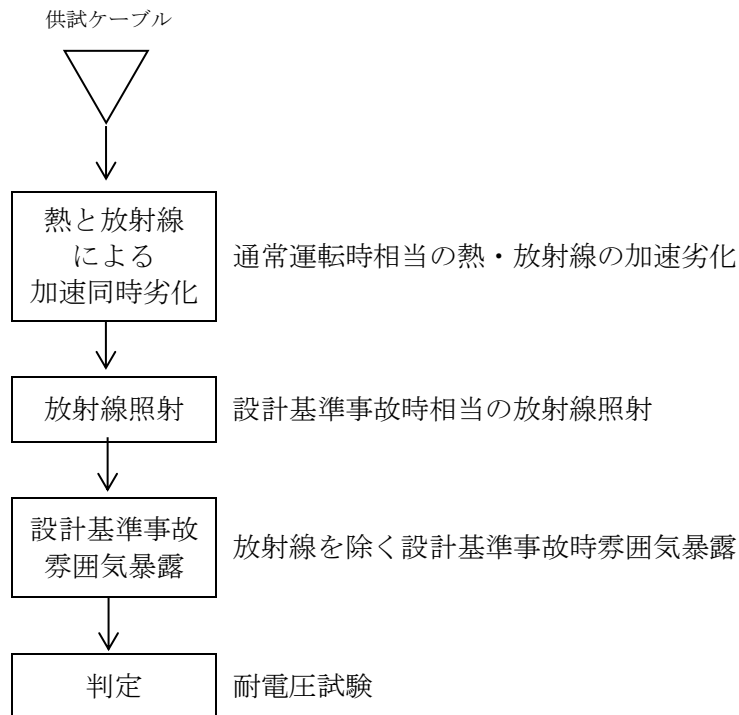
図2.9.5-3 難燃PHケーブルのACAガイドに基づく試験手順
