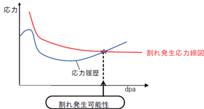
図 2.9.3-1 割れ発生予測評価概念図
