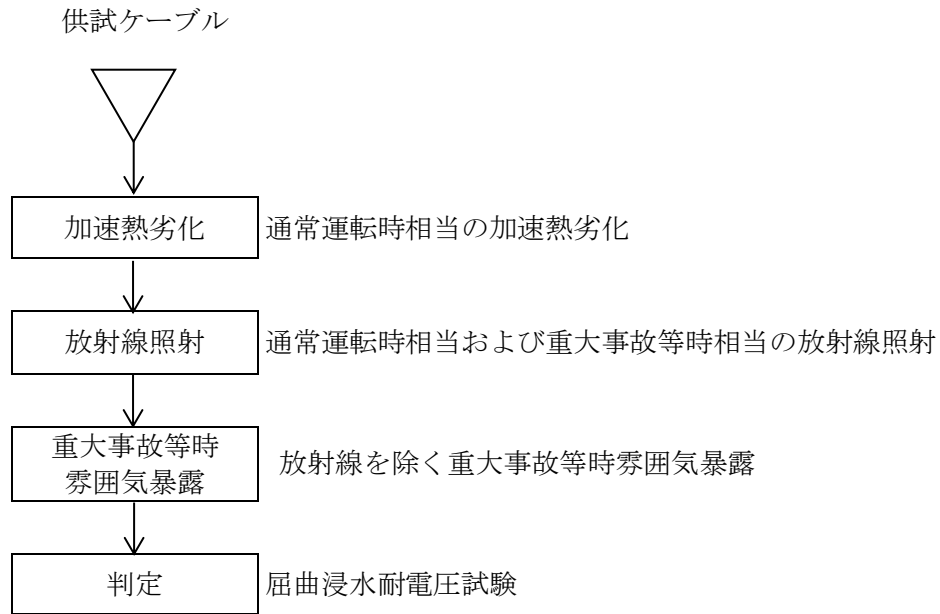
図2.9.5-4 難燃PHケーブルの長期健全性試験手順および判定方法
