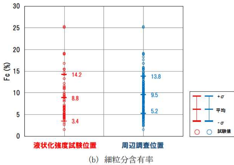
第 4.3-2 図 液化強度試験位置の基本物性の比較(1,2号埋戻土)
