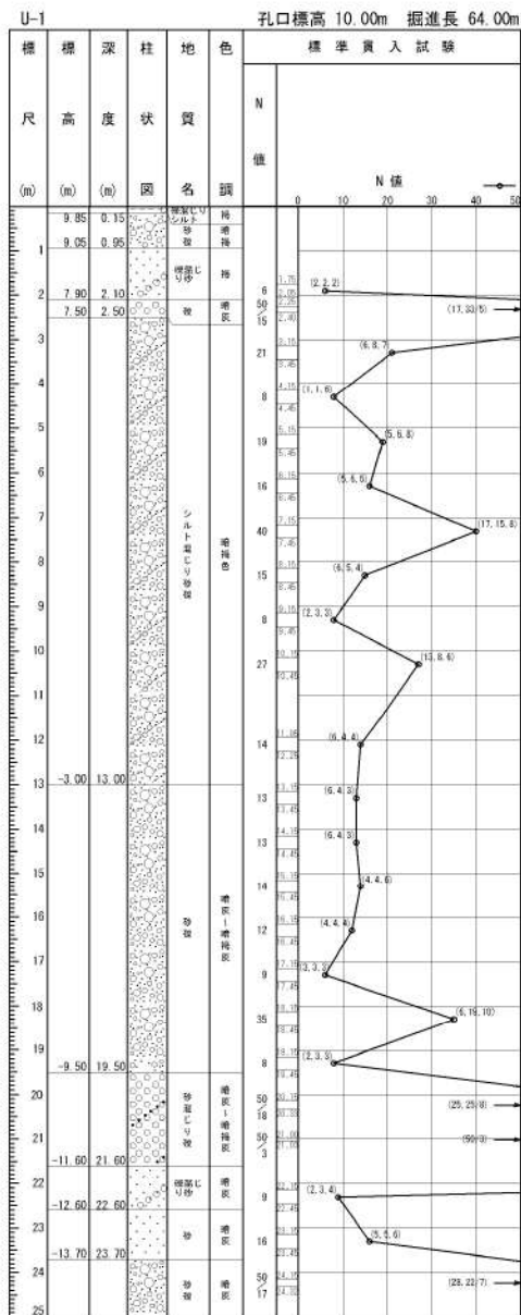
添付 1-32 図(1/3) ボーリング柱状図・コア写真 (U-1)
