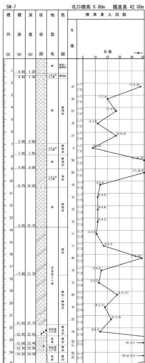
添付 1-37 図(1/2) ボーリング柱状図・コア写真 (SW-7)
