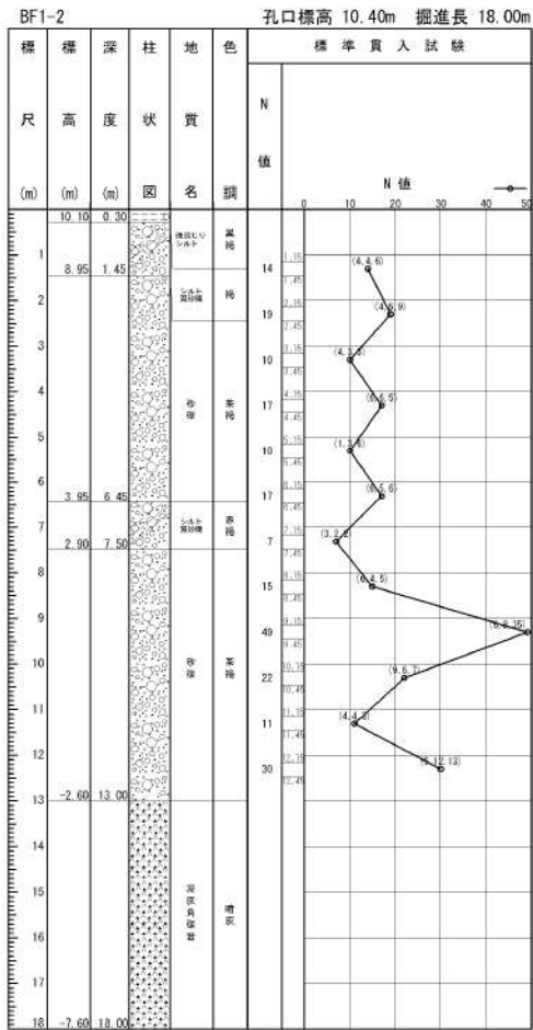
添付 1-3 図 ボーリング柱状図・コア写真 (BF1-2)
