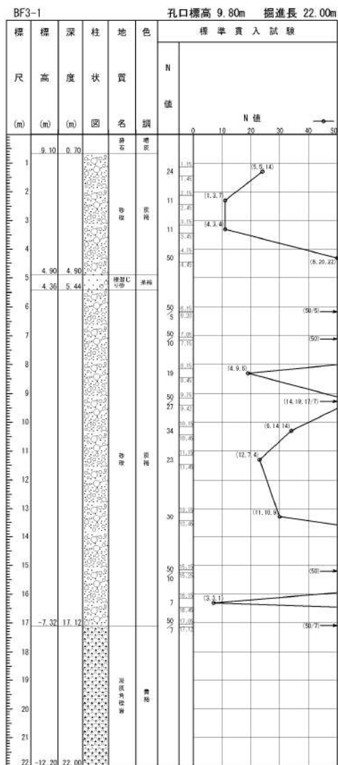
添付 1-26 図 ボーリング柱状図・コア写真 (BF3-1)
