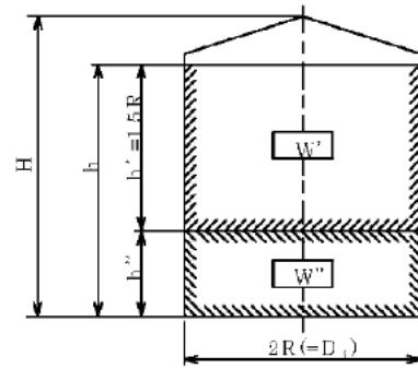
復水タンクの基礎ボルト評価に用いる 質量・高さ・径の説明図
