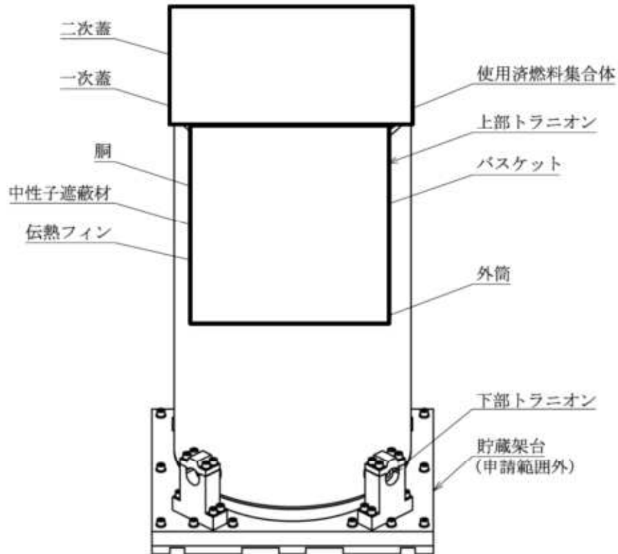
[実形状]
