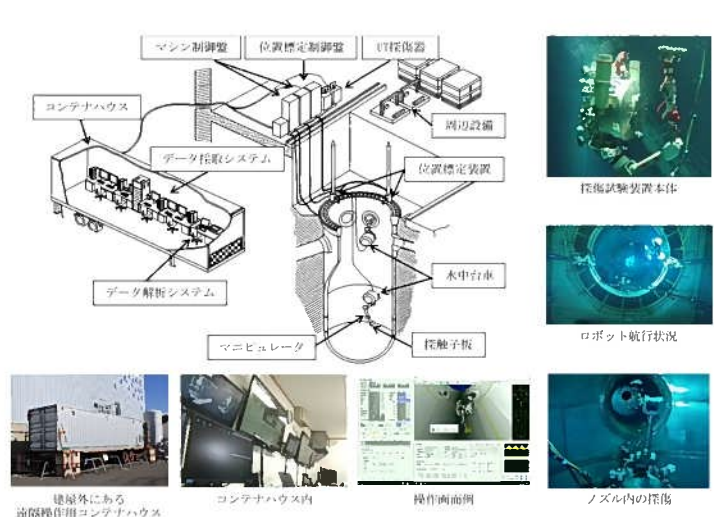
図3.1.2.2 原子炉容器超音波探傷試験装置
