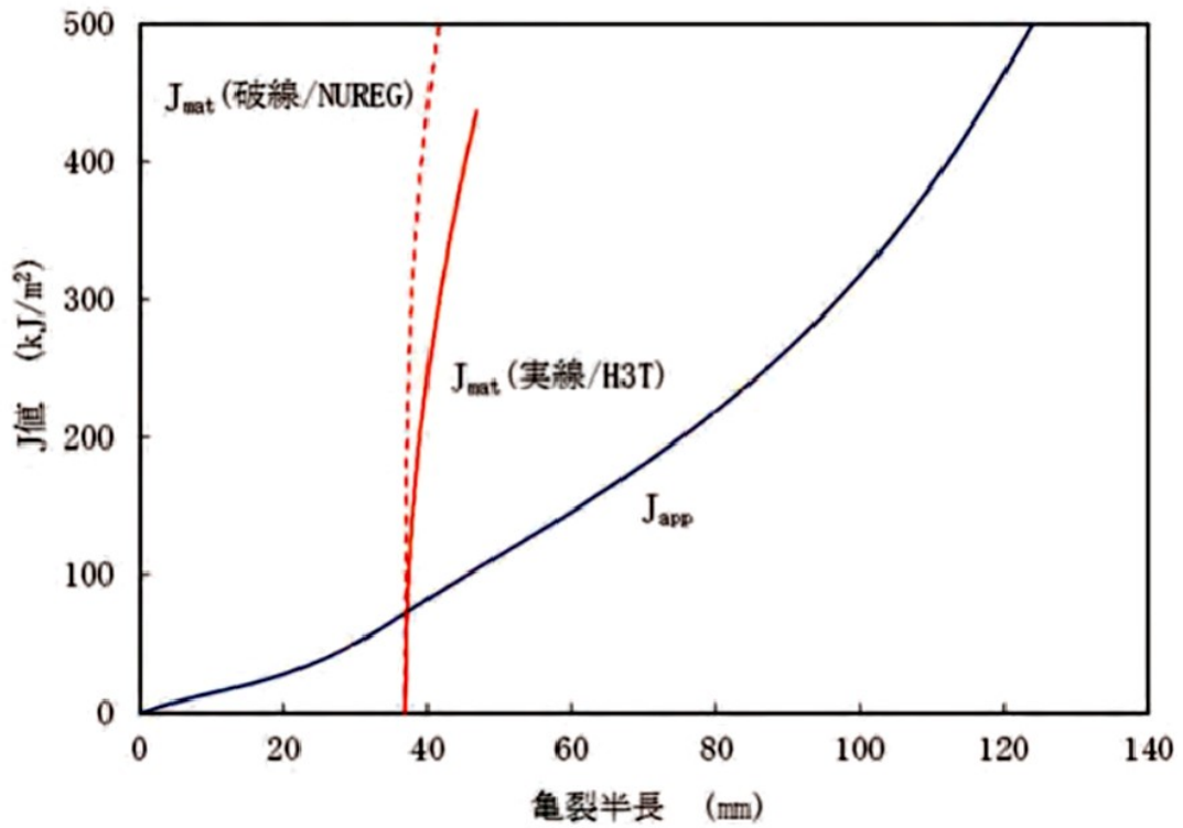
図1 ホットレグ直管
