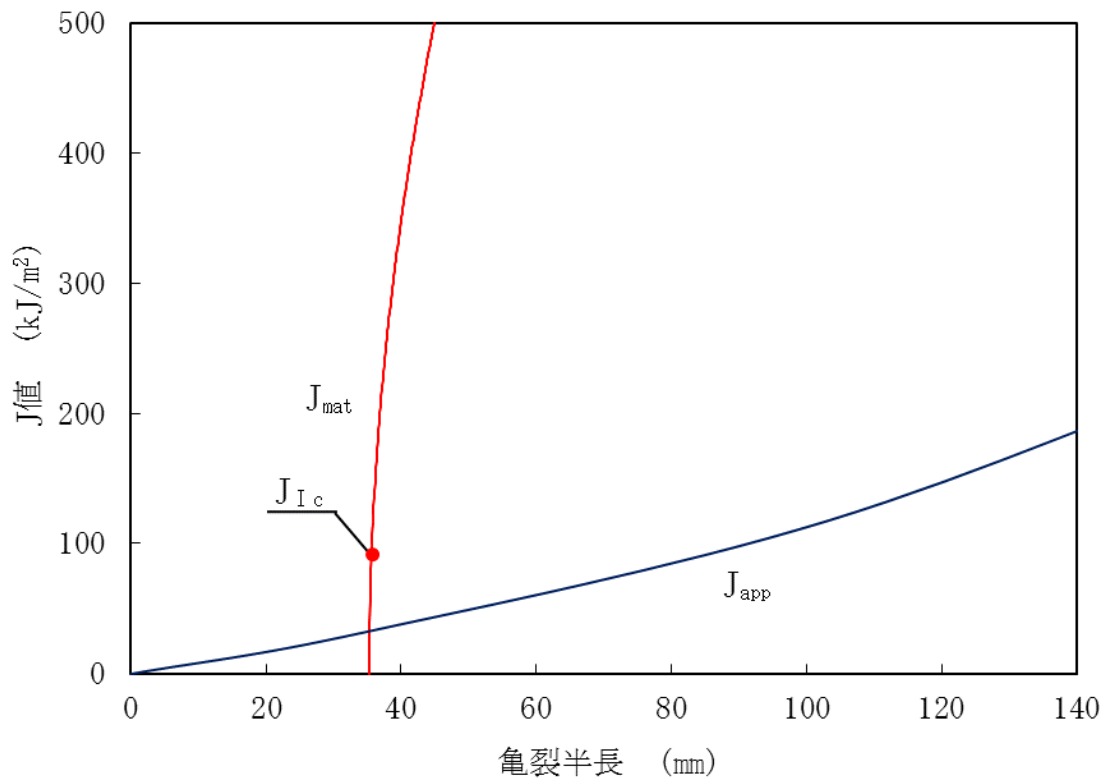
図9 RV 入口 32° エルボの亀裂安定性評価線図
