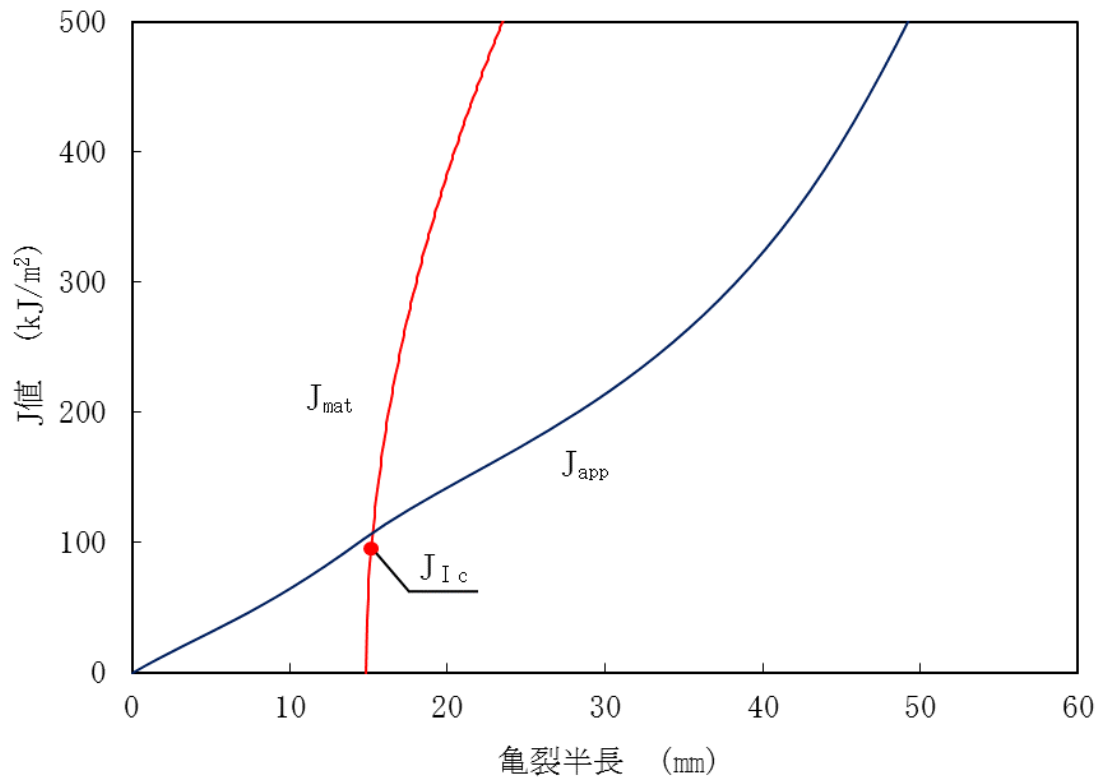
図10 蓄圧タンク注入ライン管台の亀裂安定性評価線図
