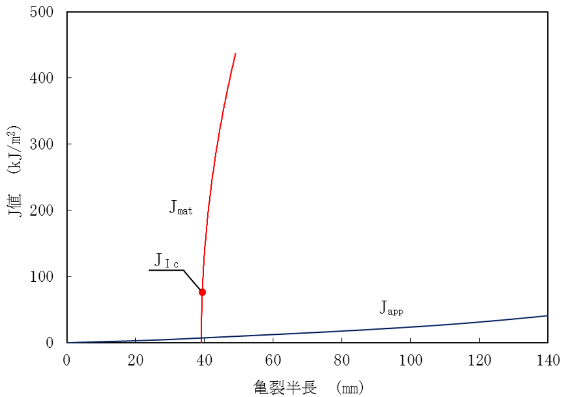
図8 クロスオーバレグ直管（垂直管）の亀裂安定性評価線図
