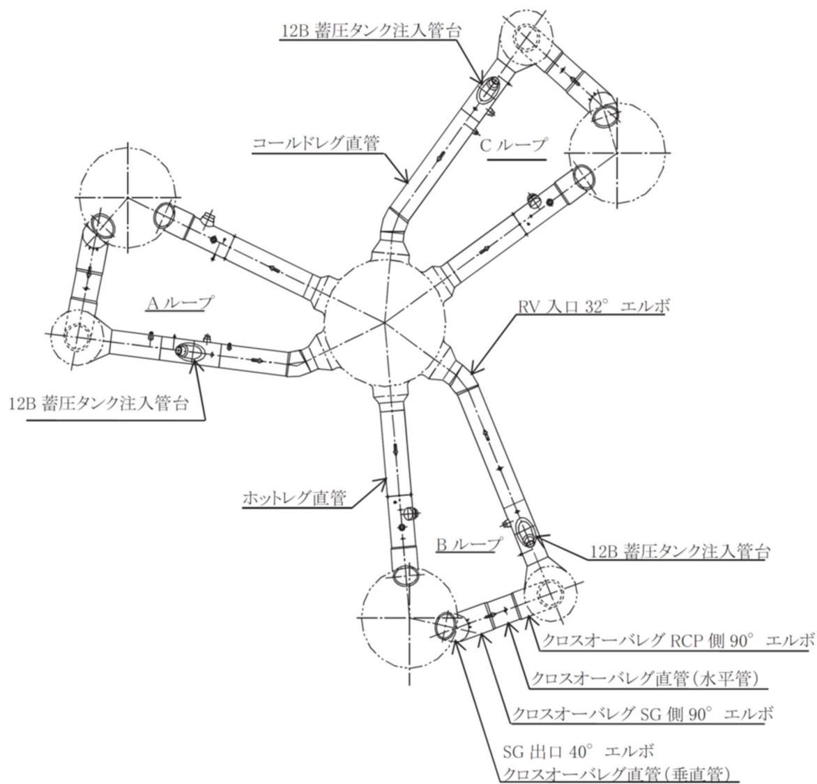
図3 1次冷却材管の熱時効評価対象部位
